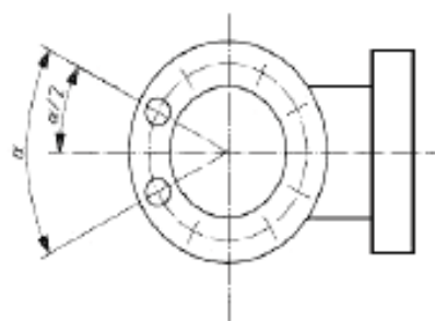
Рисунок 3 — Крестовина
