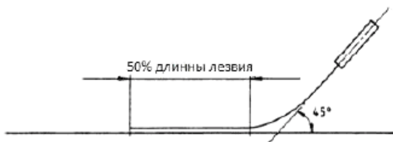
Рисунок 2 - Испытания на прочность лезвия
