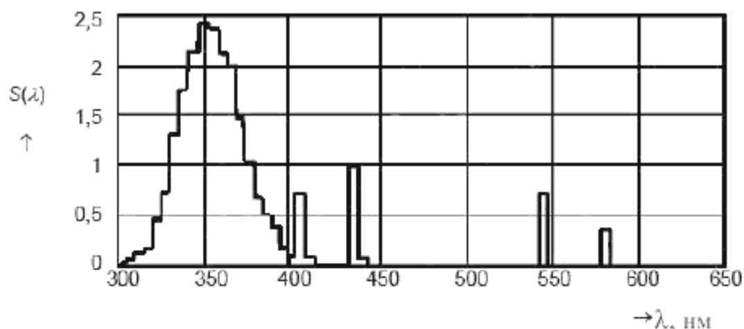
Рисунок 2 – Спектральное распределение излучения лампы
