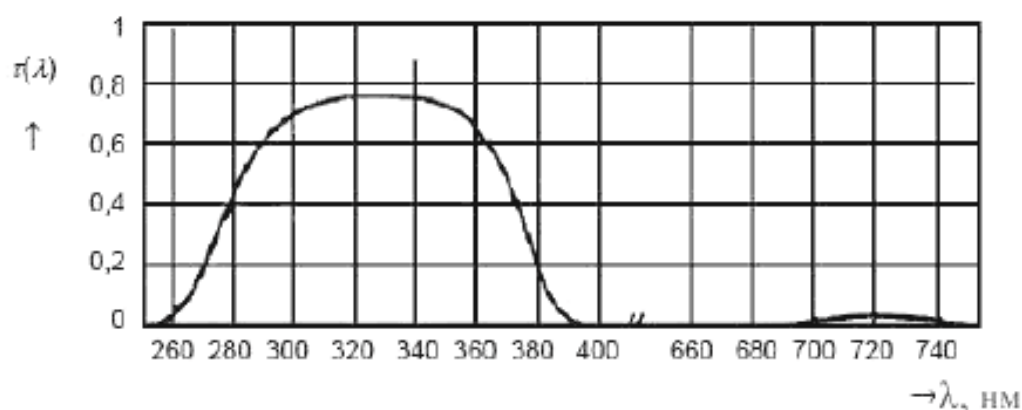
Рисунок 3 – Спектральный коэффициент пропускания \tau(\lambda) корректирующего УФ-фильтра
