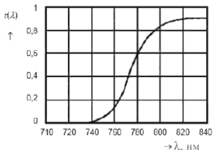
Рисунок 4 - Спектральный коэффициент пропускания \tau(\lambda) корректирующего ИК-фильтра
