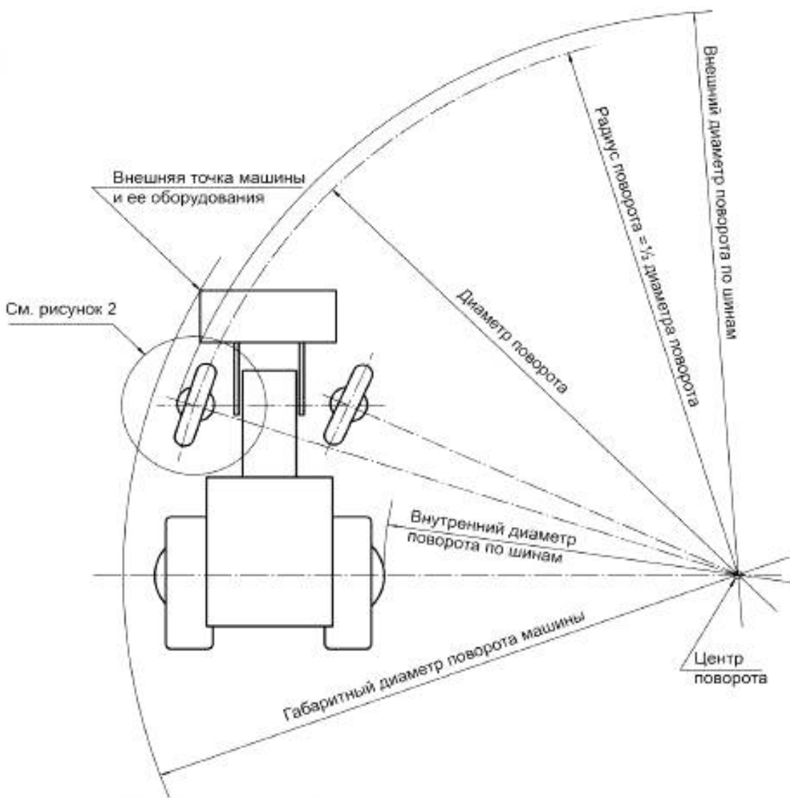
б) другие колесные машины
