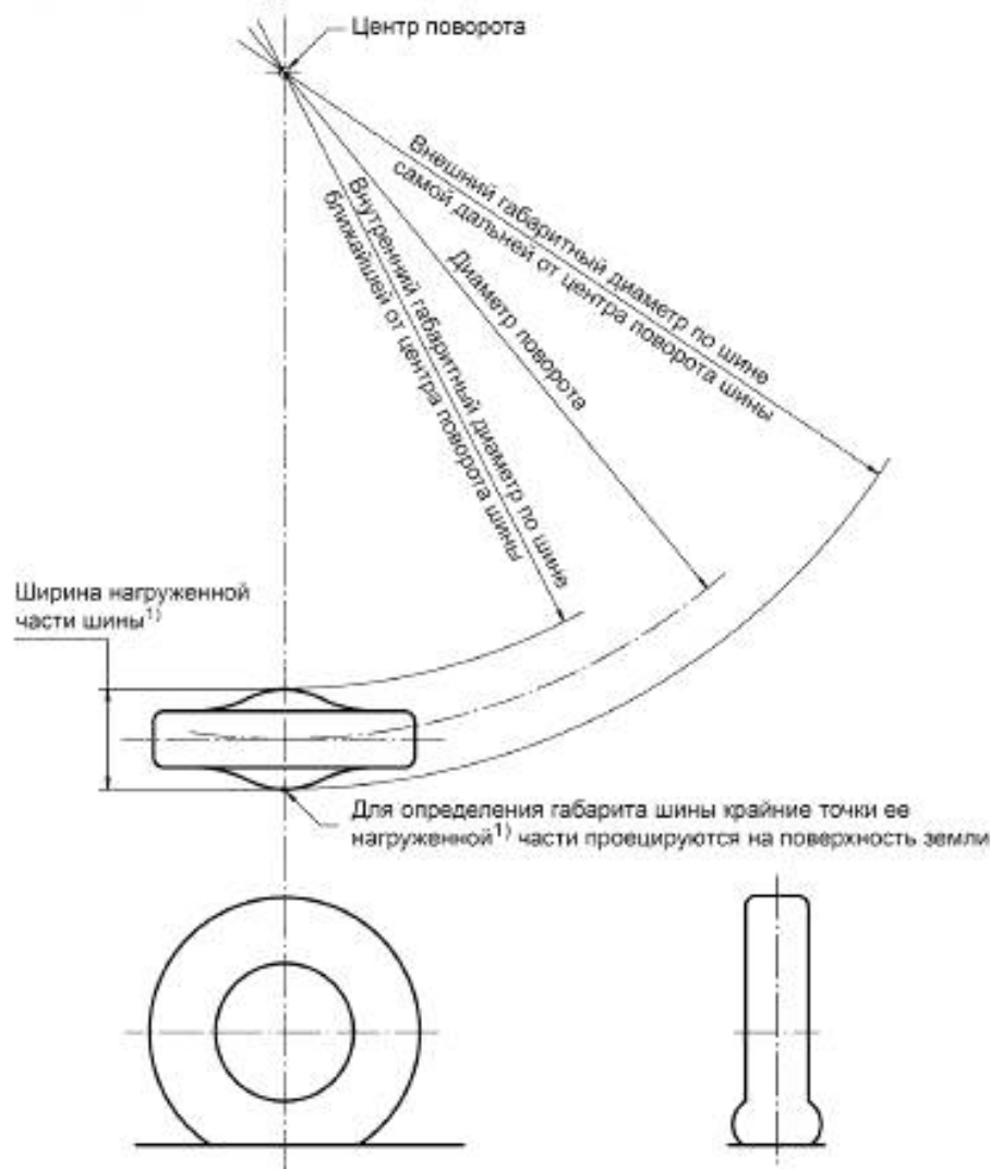
Рисунок 2 — Габаритные диаметры по шинам
