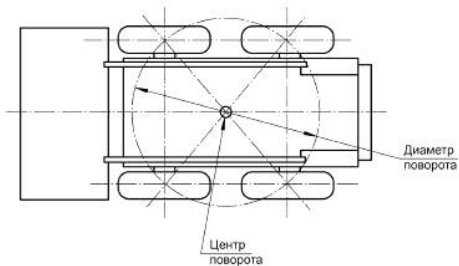
а) машина с бортовым поворотом
