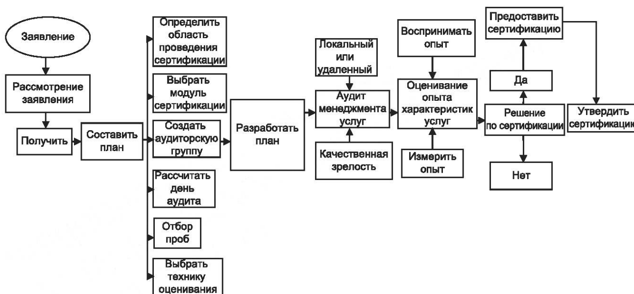
Рисунок А.1 — Блок-схема для сертификации услуг
