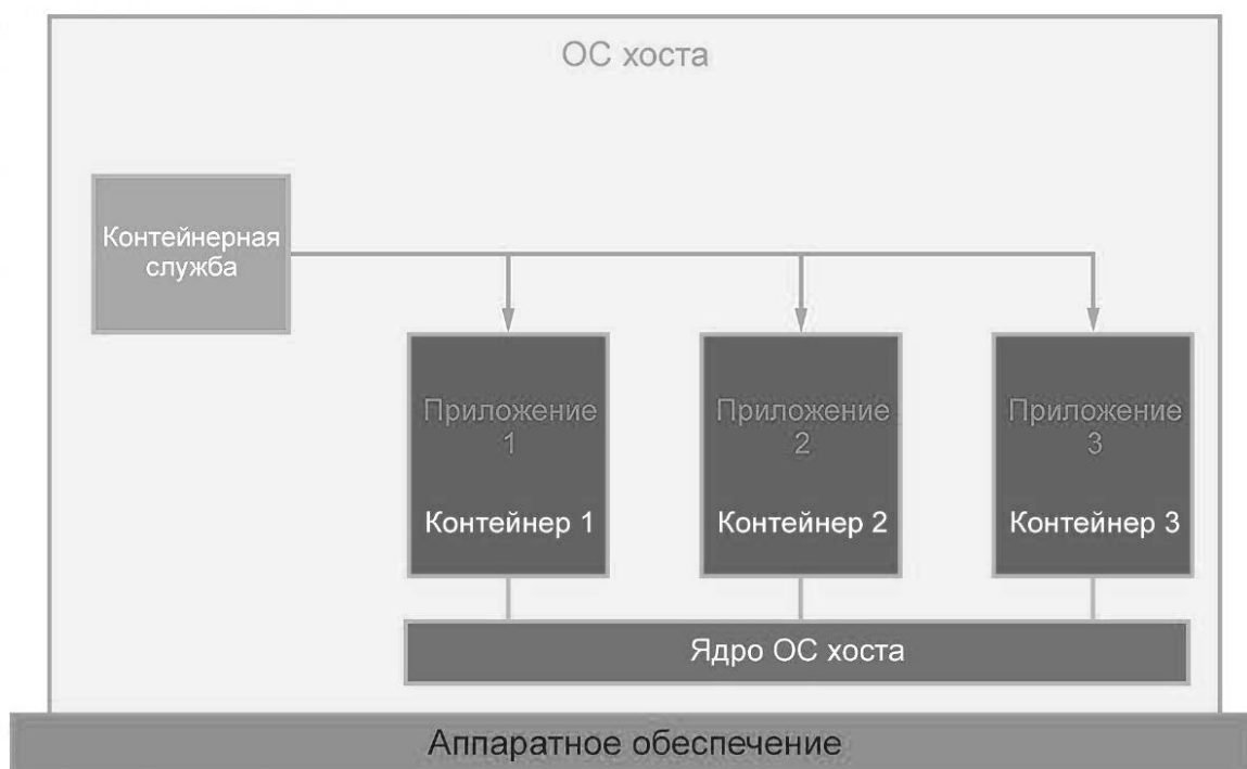
Рисунок 3 — Виртуализация контейнеров
