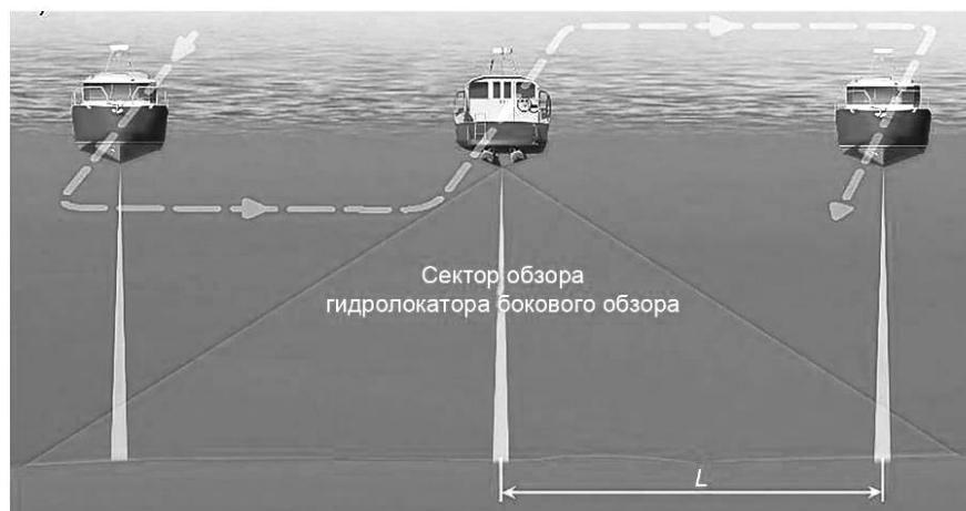
б) Промер с инструментальной оценкой рельефа дна — промер, выполняемый в сочетании с обзором дна между галсами с помощью гидролокатора бокового обзора
