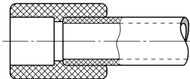
в) Соединение
