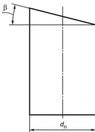
Рисунок В.2 — Конструкция сегмента
