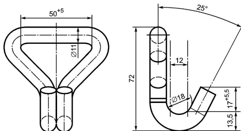
Рисунок 2 — Эталонный крюк
