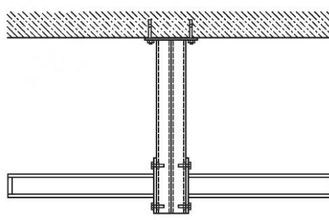
б) Двухстороннее исполнение
