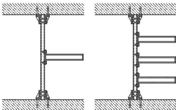
Рисунок А.3 — Двухуровневая кабельная полка, установленная с одной стороны на кабельной стойке, закрепленной к двум жестким опорам по типу «пол-потолок»
