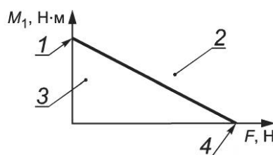
Рисунок М.2 — Графическая иллюстрация безопасных нагрузок
