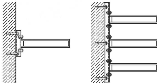
Рисунок А.2 — Двухуровневая кабельная полка, установленная на кабельной стойке, закрепленной к строительной конструкции
