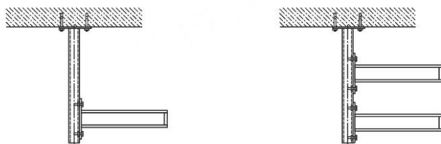
Рисунок А.5 — Двухуровневая кабельная полка, установленная с одной стороны, закрепленная на кабельной стойке при ее вертикальном подвесе с креплением к жесткой опоре по типу «потолок»
