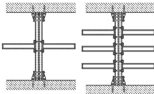
Рисунок А.4 — Двухуровневая кабельная полка, установленная с двух сторон на кабельной стойке, закрепленной к двум жестким опорам по типу «пол-потолок»
