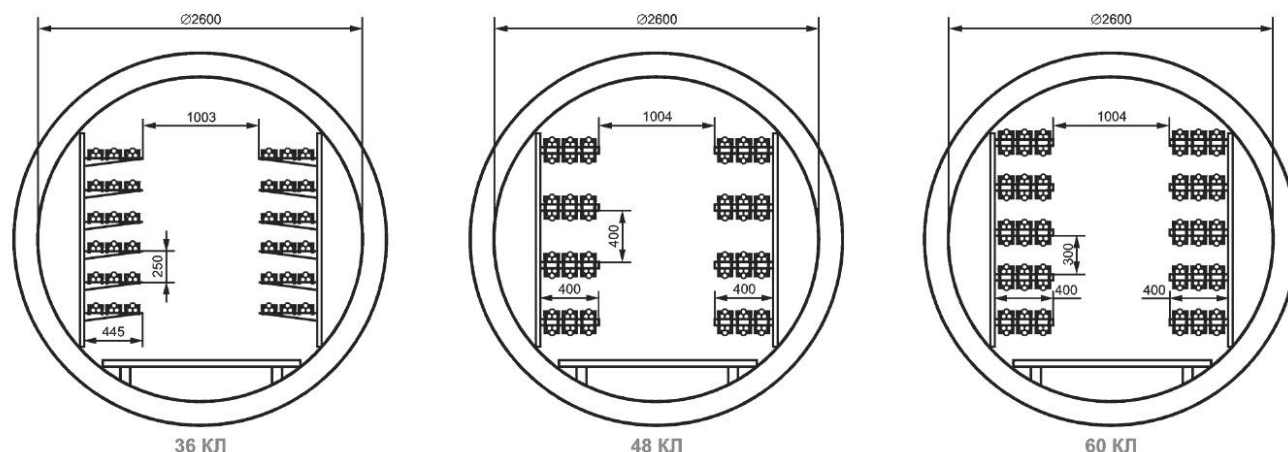
Рисунок 3 — Двухуровневая прокладка кабельных линий в кабельном коллекторе
