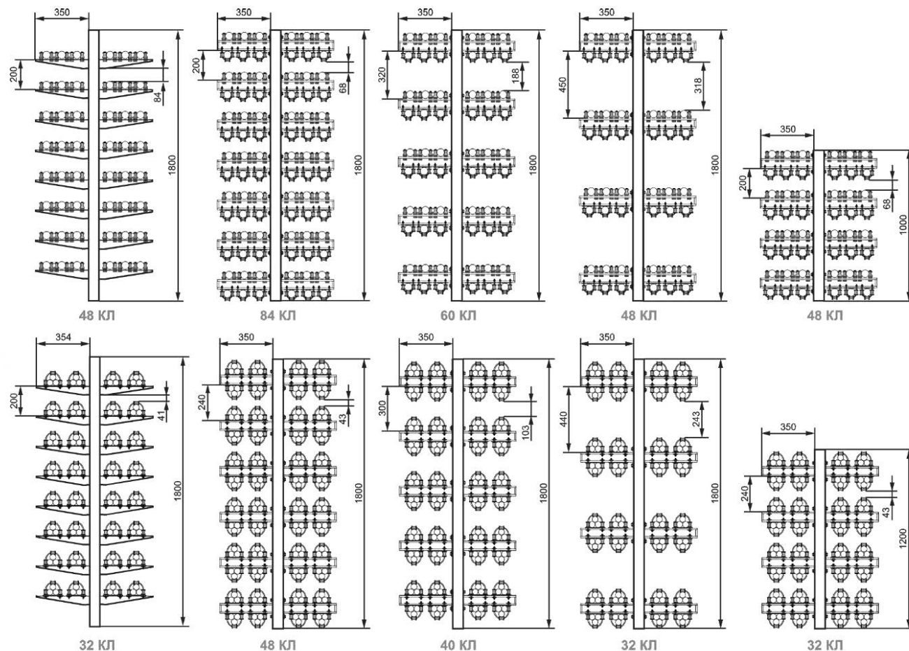
Рисунок 1 — Двухуровневая прокладка кабельных линий на кабельной эстакаде
