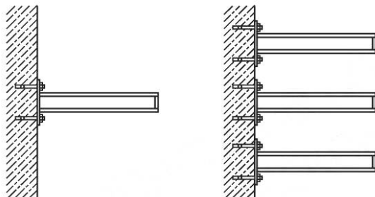
Рисунок А.1 — Двухуровневая кабельная полка, закрепленная непосредственно к опорной конструкции
