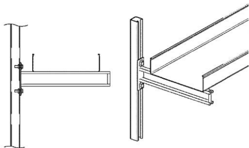
Рисунок Г.1 — Системы кабельных лотков (перфорированные и неперфорированные), расположенные на верхнем ярусе двухуровневых полок
