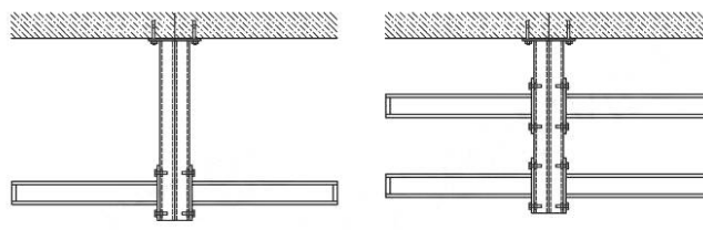
Рисунок А.6 — Двухуровневая кабельная полка, установленная с двух сторон, закрепленная на кабельной стойке при ее вертикальном подвесе с креплением к жесткой опоре по типу «потолок»
