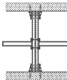
б) Двухстороннее исполнение
