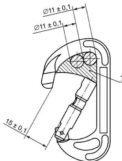
1 — зона размещения стержня (стержней)
