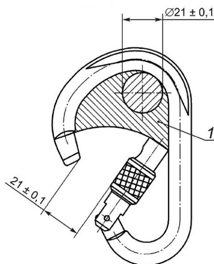
1 — зона размещения стержня
