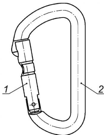
Рисунок 1 — Базовый карабин (класс В)
