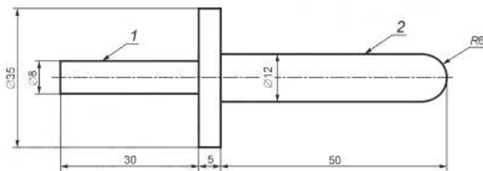
Рисунок 105 — Испытательный щуп «а»
