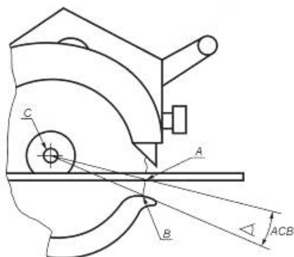
Рисунок 111 — Доступ к передней зоне зубчатого венца
