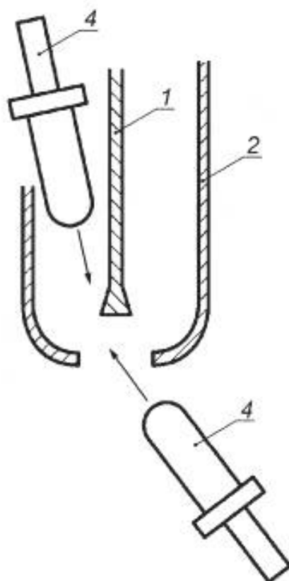
а) Пила с нижним защитным кожухом
