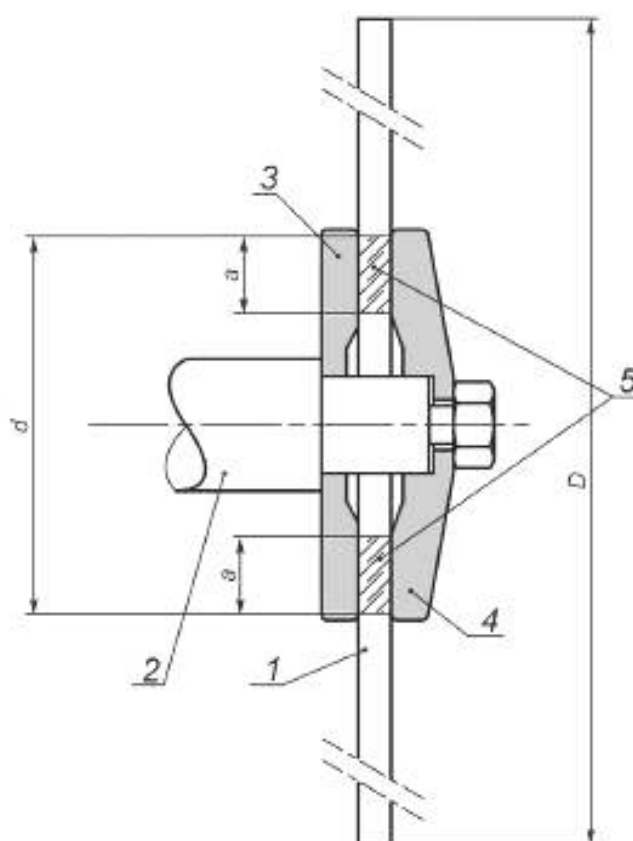
Рисунок 113 — Основные размеры опорной плиты
