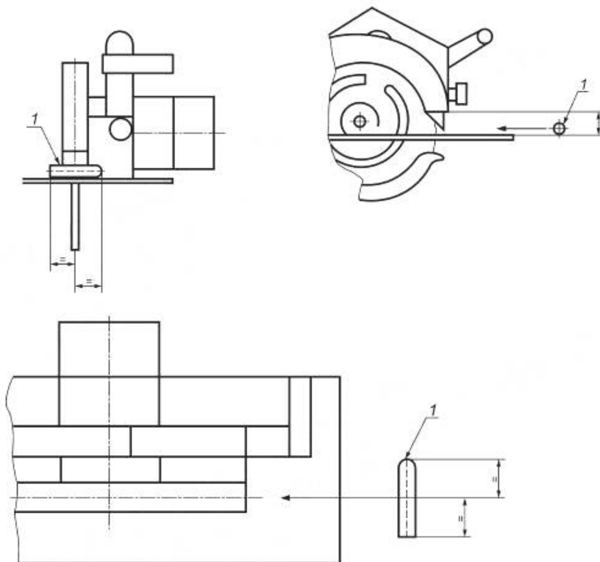
Рисунок 111 — Доступ к передней зоне зубчатого венца
