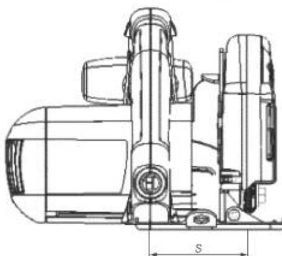
Рисунок 108с — Ограничение высоты проема. Размер S
