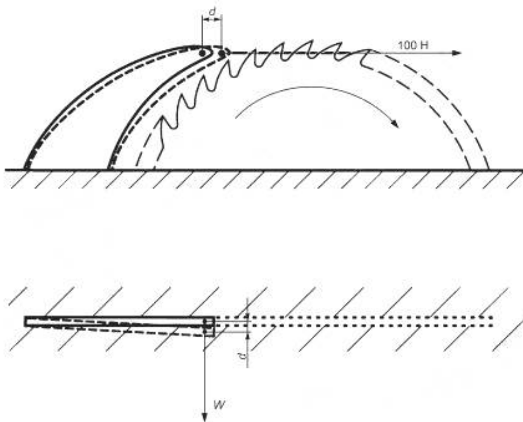
Рисунок АА.101 — Испытание устойчивости расклинивающего ножа
