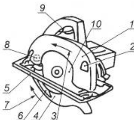
Рисунок 101 — Дисковая пила с наружным качающимся защитным кожухом
