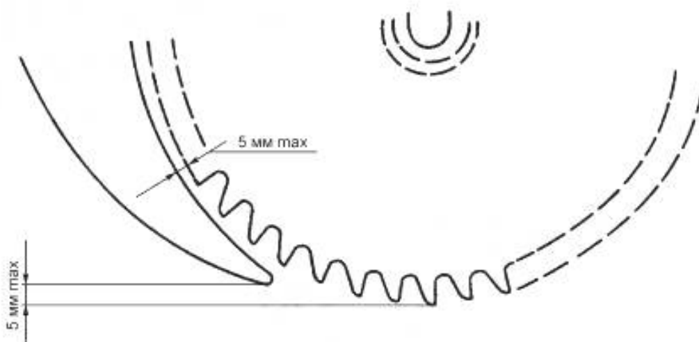
Рисунок АА.102 — Регулировка расклинивающего ножа
