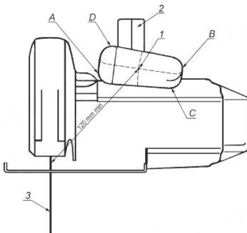
Рисунок 107а) — Дисковая пила с дополнительной рукояткой
