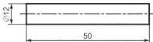
Рисунок 110 — Испытательный щуп «b»
