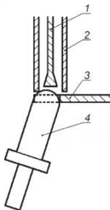
с) Врезная пила без свеса
