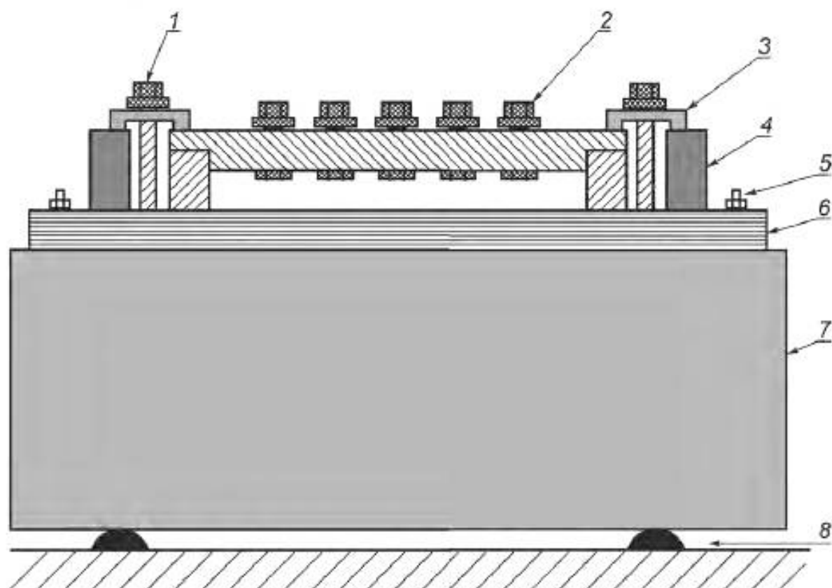
Рисунок I.103 — Место установки преобразователей для ударных гайковертов
