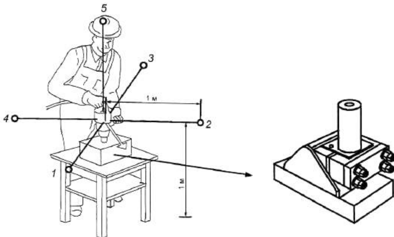
Рисунок I.101 — Тормозное устройство
