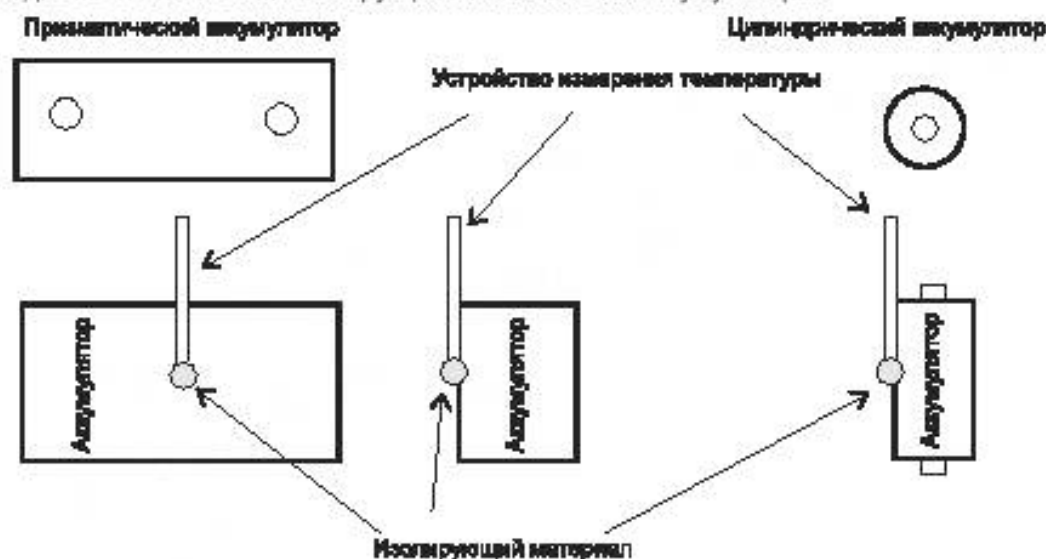
Рисунок 1 — Примеры измерения температуры аккумуляторов
