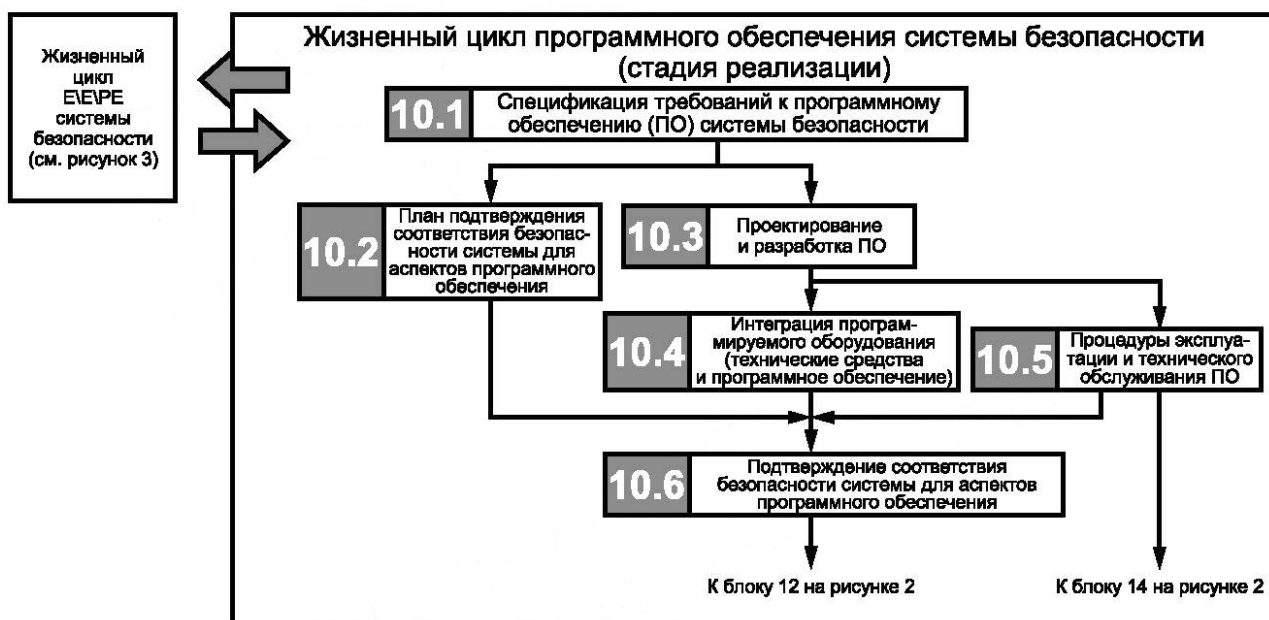
Рисунок 4 — Структура жизненного цикла программного обеспечения системы безопасности (стадия реализации)
