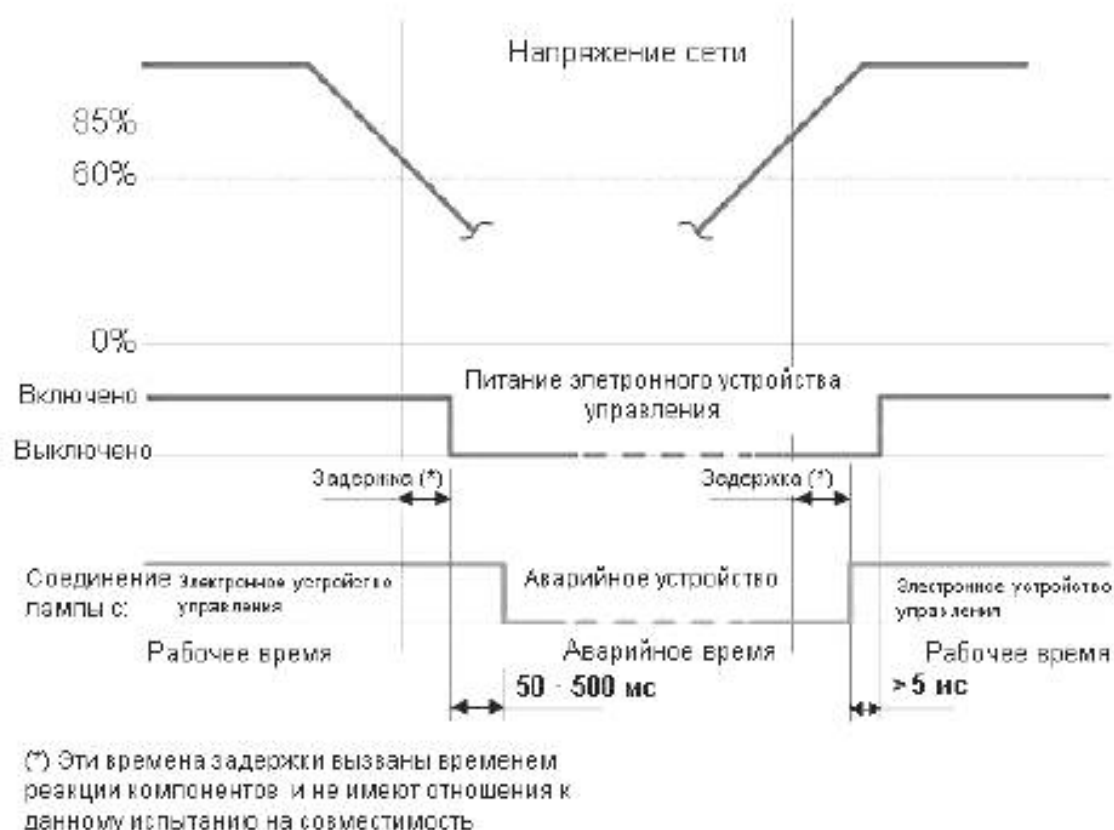
Рисунок L.1 – Временная диаграмма операции переключения
