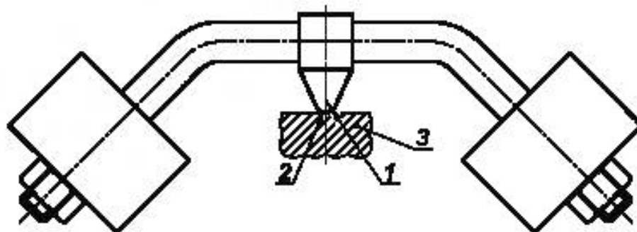
1 — R = 2,5 мм; 2 — сферический; 3 — образец
