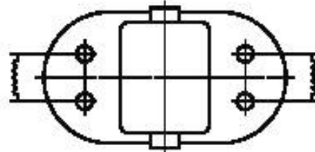
Цоколь GX32q
