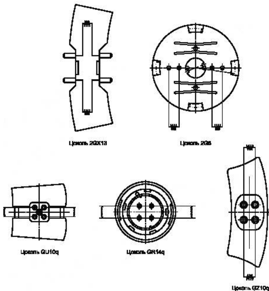
Рисунок Е.1 — Места присоединения электродов различных цоколей
