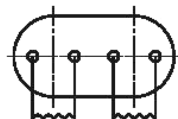
Цоколь 2G11
