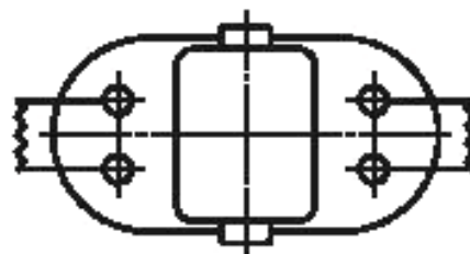
Цоколь GCS2q
