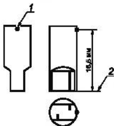
1 — точка измерения, 2 — базовая плоскость
