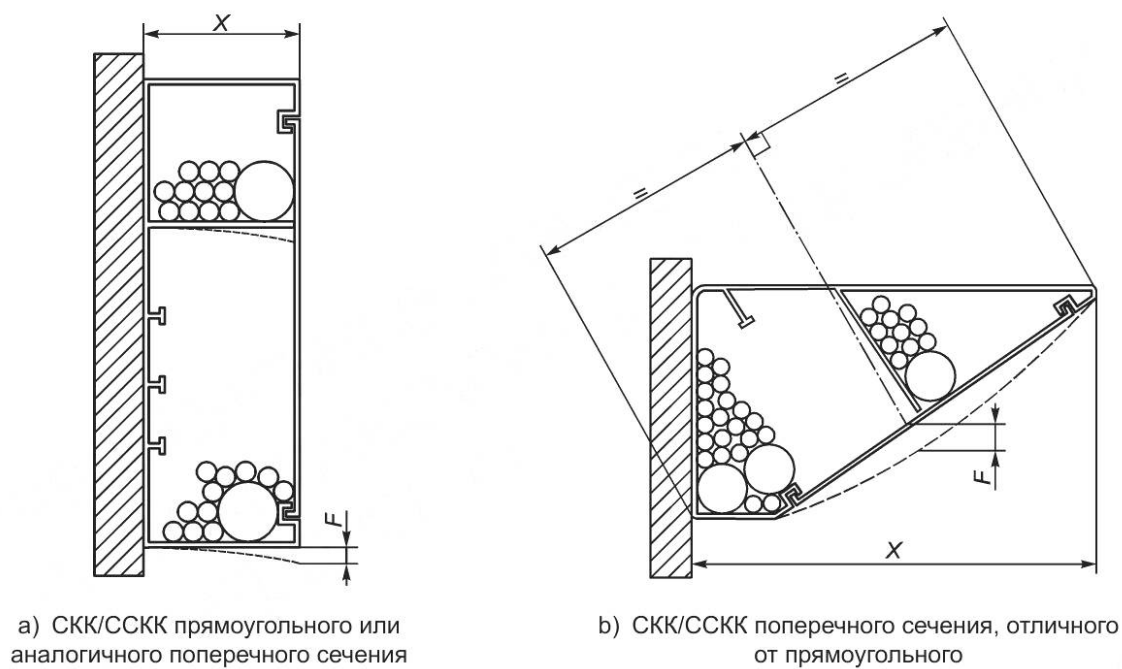
Рисунок 102 — Схема для испытания на удержание кабелей в соответствии с 10.2.2
