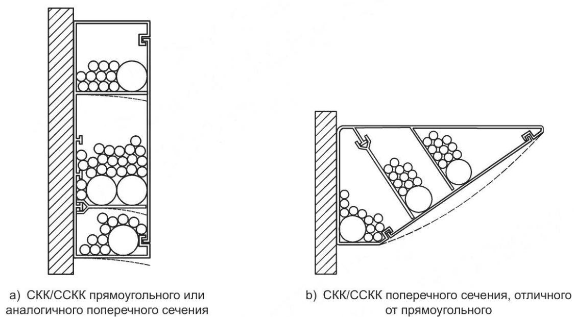
Рисунок 103 — Схема для испытания на удержание кабелей в соответствии с 10.2.3
