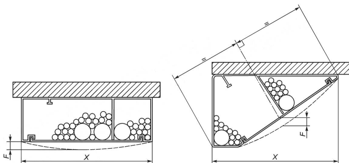
а) СКК/ССКК прямоугольного или аналогичного поперечного сечения
