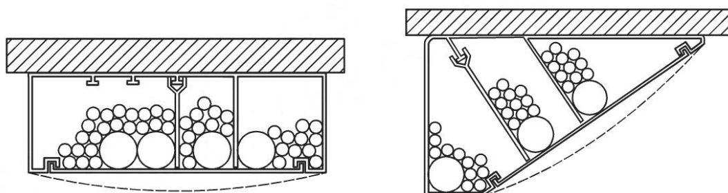
а) СКК/ССКК прямоугольного или аналогичного поперечного сечения
