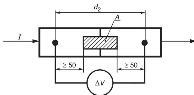
A — зона соединения; \Delta V — падение напряжения; I — ток; d_2 — расстояние между двумя точками измерения б) Схема стыкового соединения
