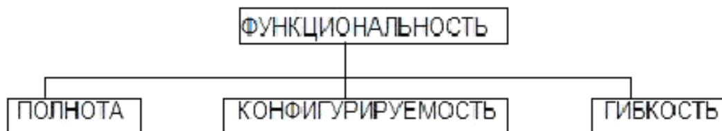
Рисунок 2 — Иерархия функциональности
