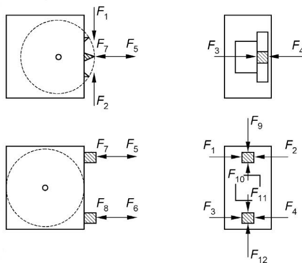
Рисунок 3e — Диск
