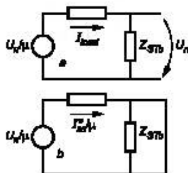
Рисунок E.5 — Учет загрузки сети
