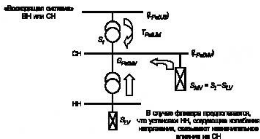
Рисунок 3 — Пример системы для разделения общих вкладов при среднем напряжении
