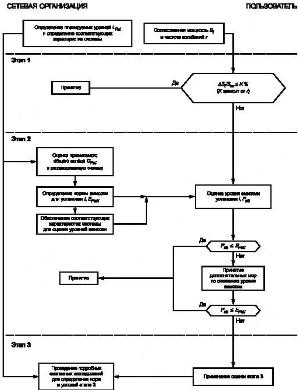
Рисунок 4 — Схема процедуры оценки
