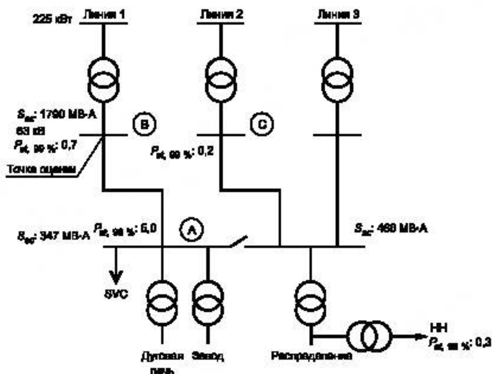
Рисунок G.4 — Нормальная конфигурация системы
