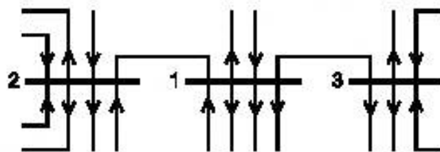
Рисунок 6 — Определение S_i для ячейистой системы ВН или СВН
