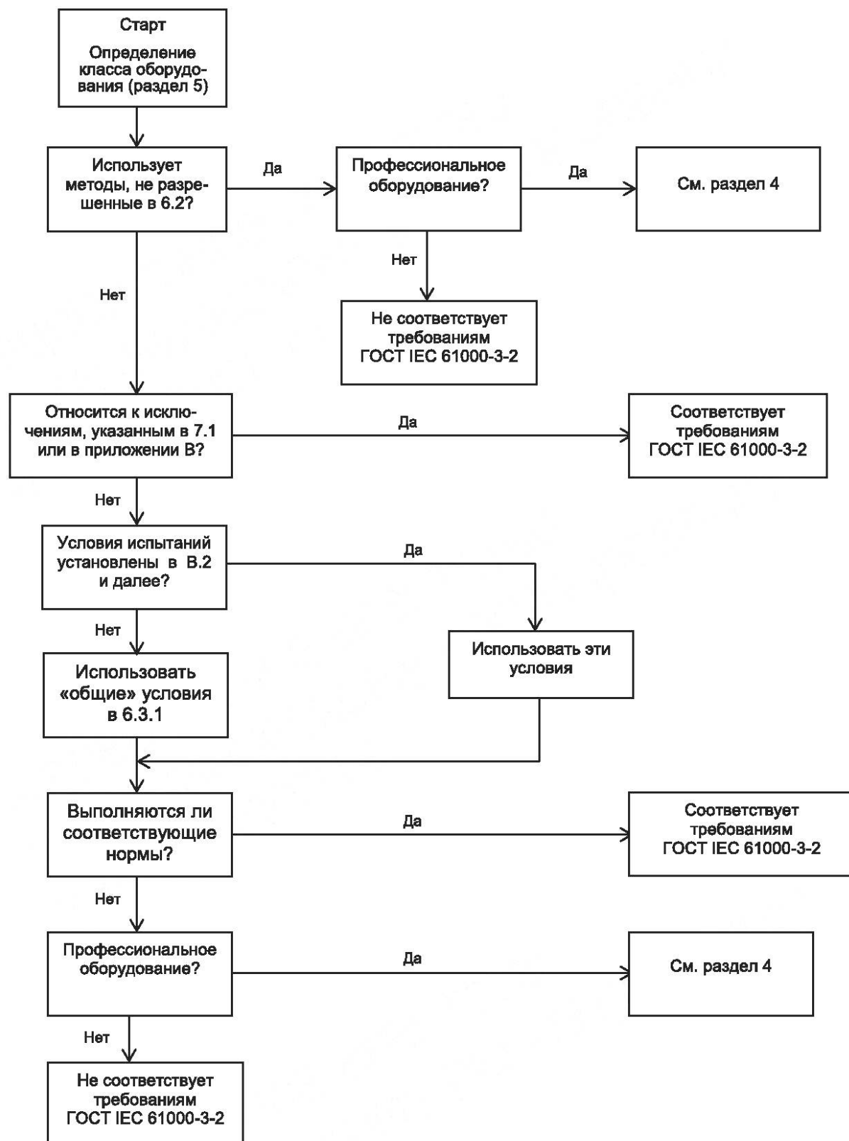
Рисунок 1 – Алгоритм для определения соответствия
