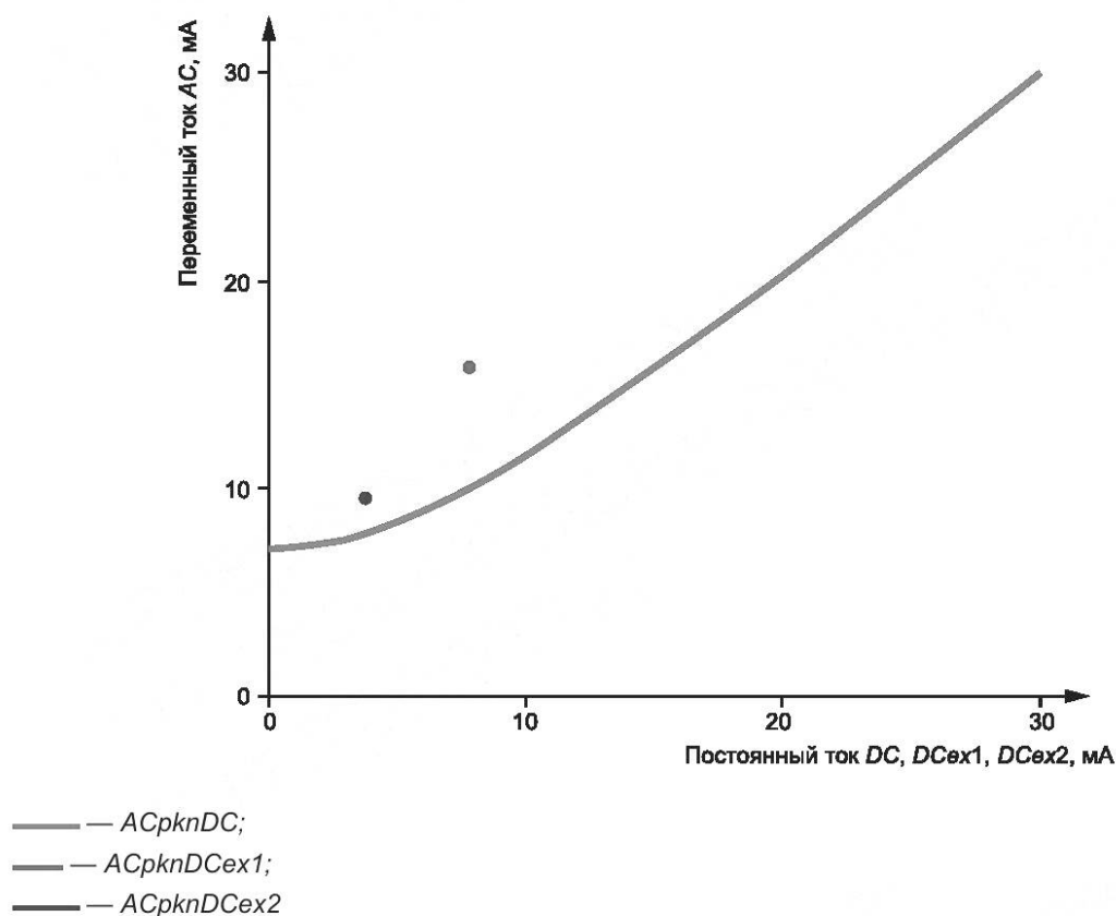
Рисунок Н.9 — Пороговое значение тока отпущения иммобилизации для комбинаций переменного и постоянного тока в соответствии с IEC TS 60479-2 с дополнительными данными
