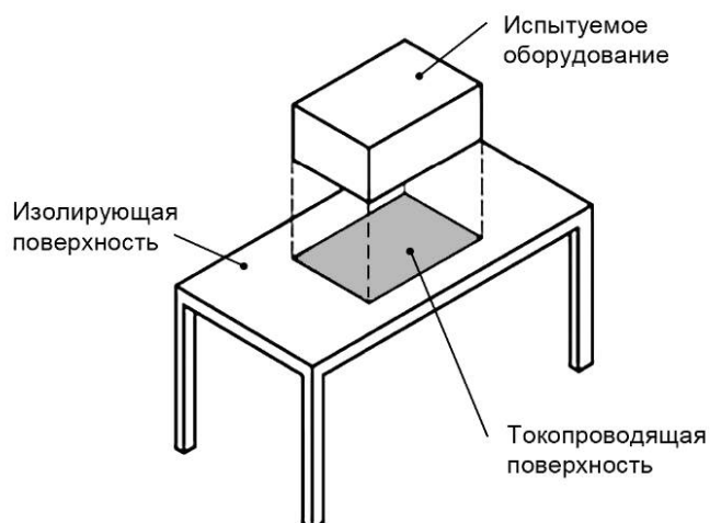
Рисунок В.1 — Рабочая площадка для оборудования
