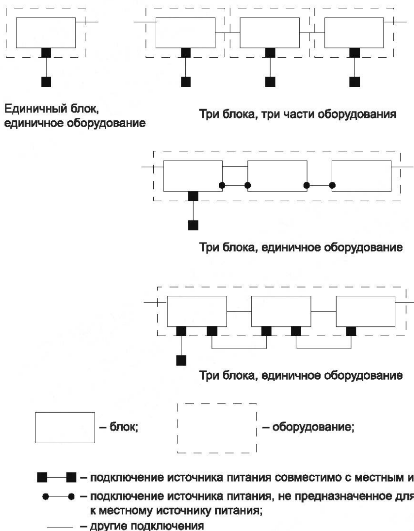
Рисунок А.1 — Оборудование
