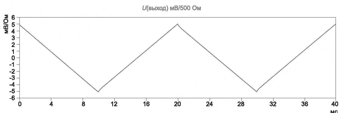
Рисунок Н.2 — Треугольная форма сигнала ТОКА ПРИКОСНОВЕНИЯ для схемы отпускания иммобилизации
