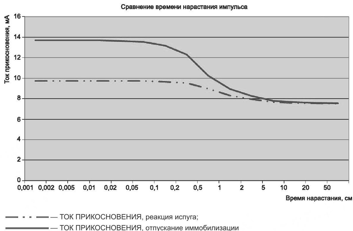
Рисунок Н.5 — График зависимости ТОКА ПРИКОСНОВЕНИЯ от времени нарастания для сигнала длительностью 20 мс прямоугольной формы
