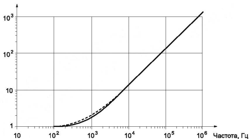
Частотный коэффициент
