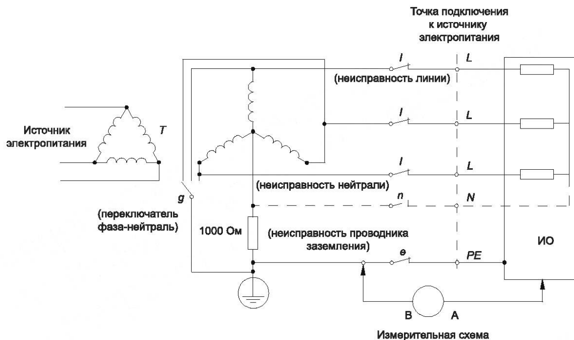
Рисунок 12 — Трехфазное оборудование в системе IT с соединением звездой
