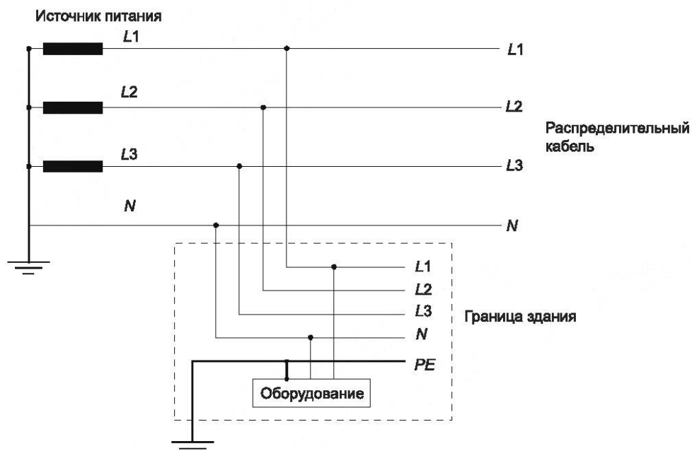
Рисунок I.5 — Пример трехфазной системы энергообеспечения TT с нейтралью
