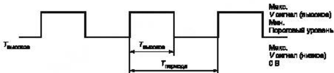
Рисунок E.5a — Типичный ШИМ-сигнал
