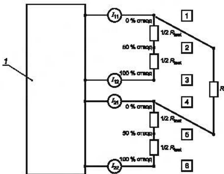
1 — испытуемый ЭПРА; R_L — резистор, заменяющий лампу; I_{on} — измеряемый ток; 1...6 — положения переключателя
