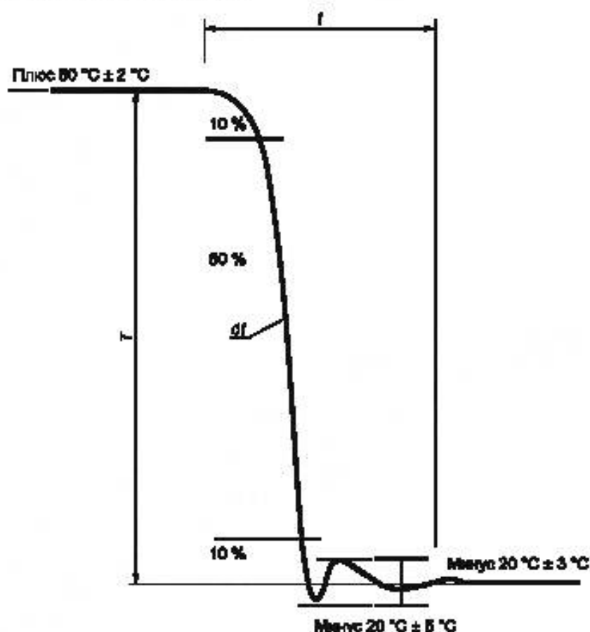
Рисунок 5 — Пример циклического воздействия температуры, описанного в 15.2 d) 2)
