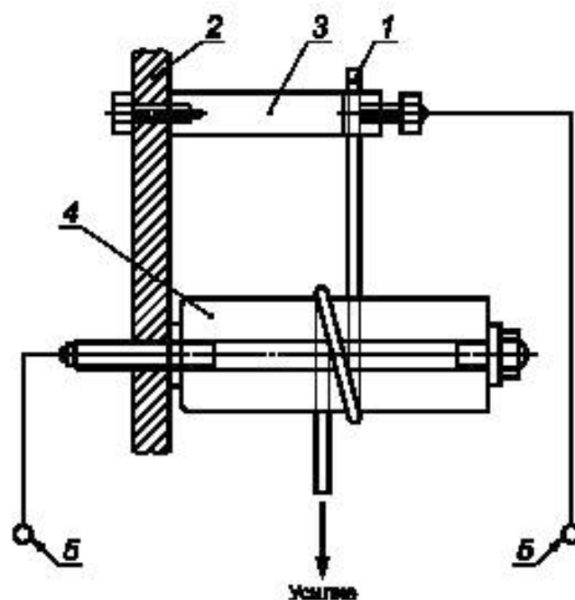
1 — образец; 2 — изоляционный материал; 3 — верхний зажим; 4 — цилиндр; Б — испытательное напряжение
