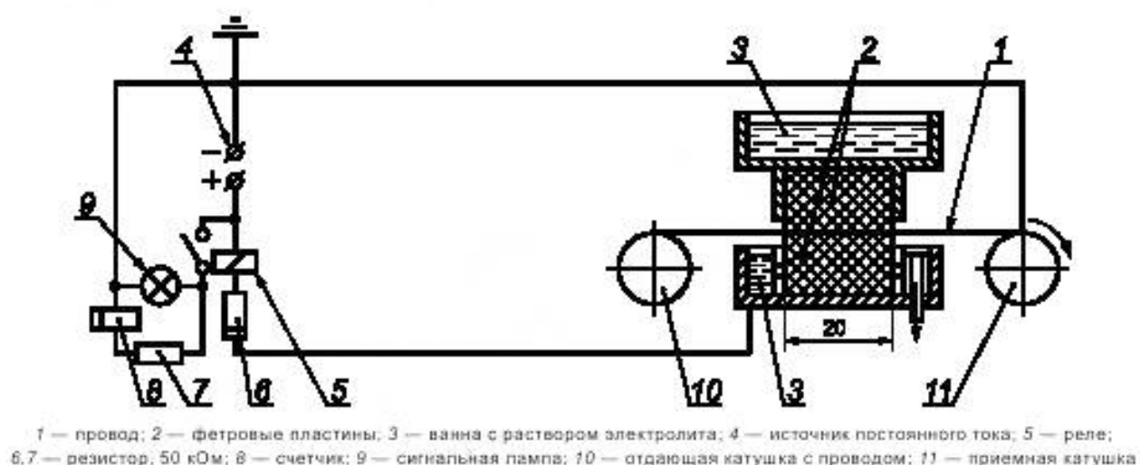
Рисунок 5 — Схема установки для определения числа точечных повреждений при низком напряжении
