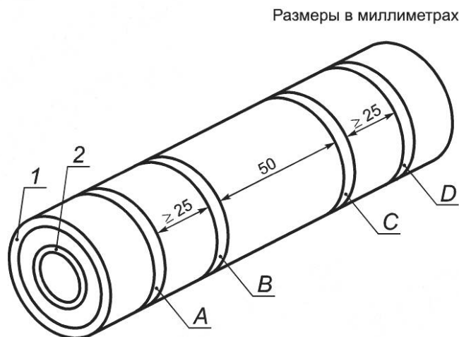
а) Образец для измерений удельного объемного электрического сопротивления экрана по жиле
