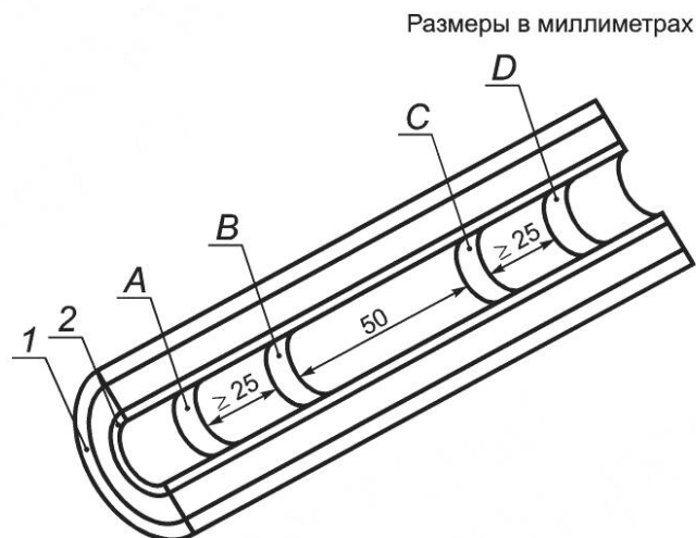
а) Образец для измерений удельного объемного электрического сопротивления экрана по жиле
