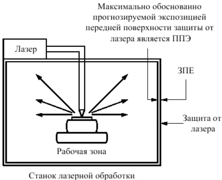
Рисунок С.1 – Пример защиты вокруг станка лазерной обработки
