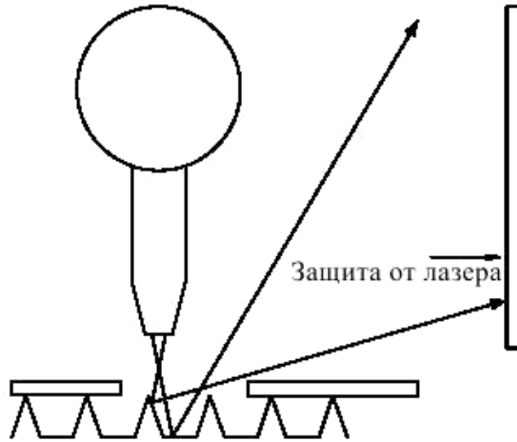
Рисунок В.3с – Отсутствие заготовки
