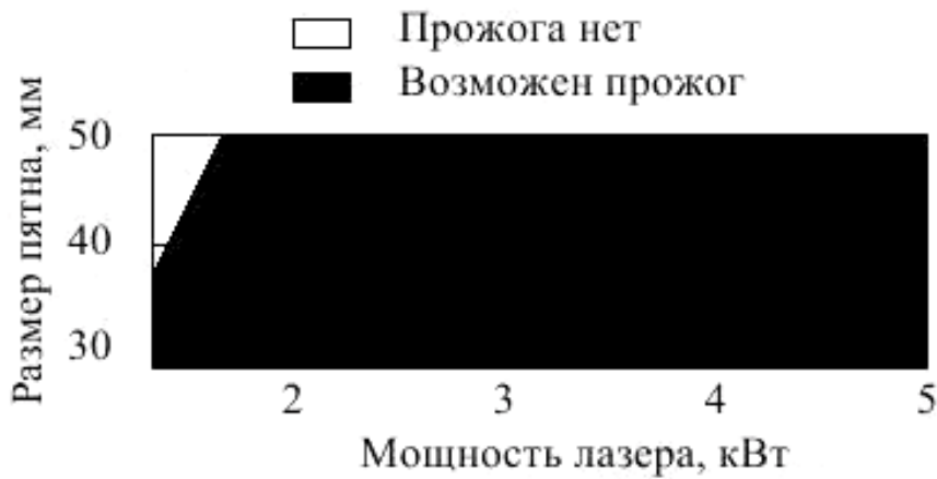
Рисунок F.12 – Стойкость к разрушению листа поликарбоната толщиной 6 мм от 100 с экспозиции расфокусированного пучка во время экспериментов с использованием непрерывного лазера на углекислом газе
