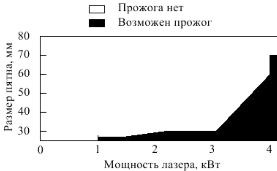
Рисунок F.13 – Стойкость к разрушению листа оцинкованной стали толщиной 1 мм от 10 с экспозиции расфокусированного пучка во время экспериментов с использованием непрерывного лазера на иттрий-алюминиевом гранате с неодимом
