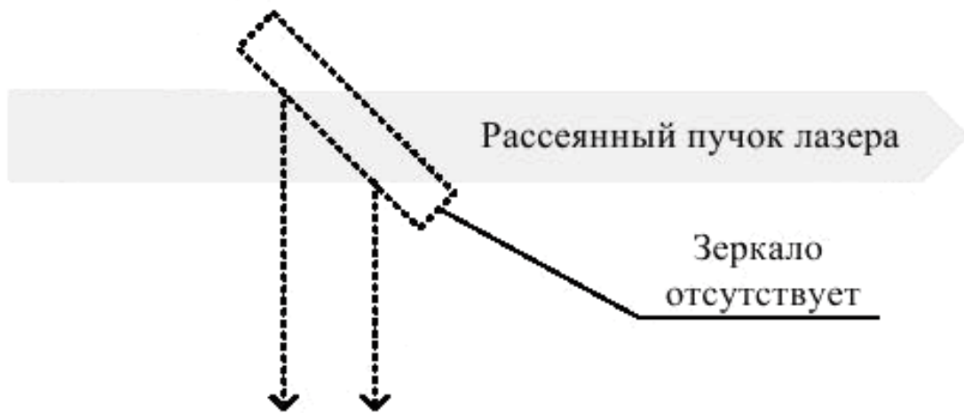
Рисунок В.4а – Работа лазера при отсутствии поворачивающего зеркала
