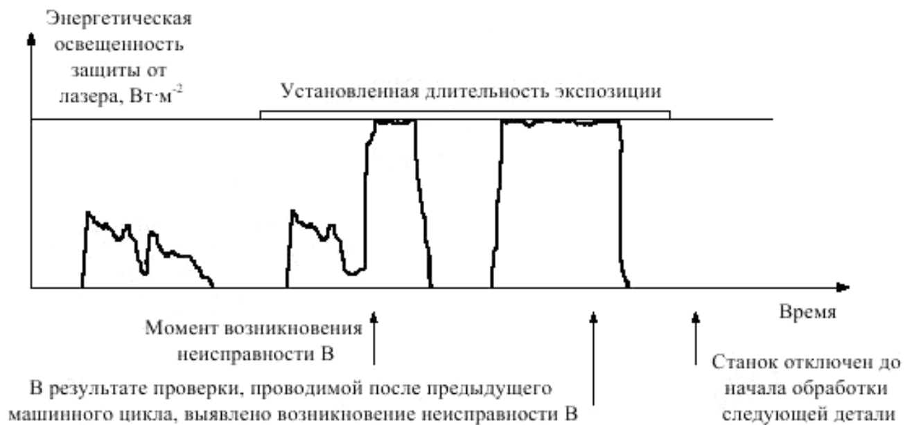
Рисунок В.6б – Отключение лазера при использовании автономного машинного мониторинга безопасности
