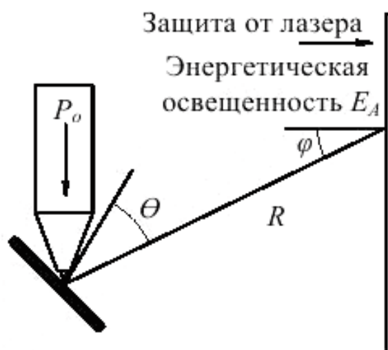
Рисунок В.1 – Расчет диффузного отражения
