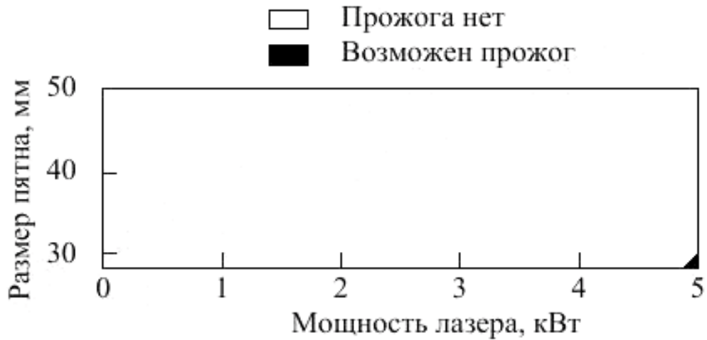
Рисунок F.11 – Стойкость к разрушению листа поликарбоната толщиной 6 мм от 10 с экспозиции расфокусированного пучка во время экспериментов с использованием непрерывного лазера на углекислом газе
