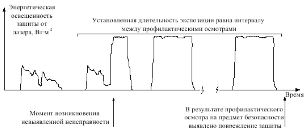
Рисунок В.7 – Установленная длительность экспозиции для станков без системы мониторинга безопасности
