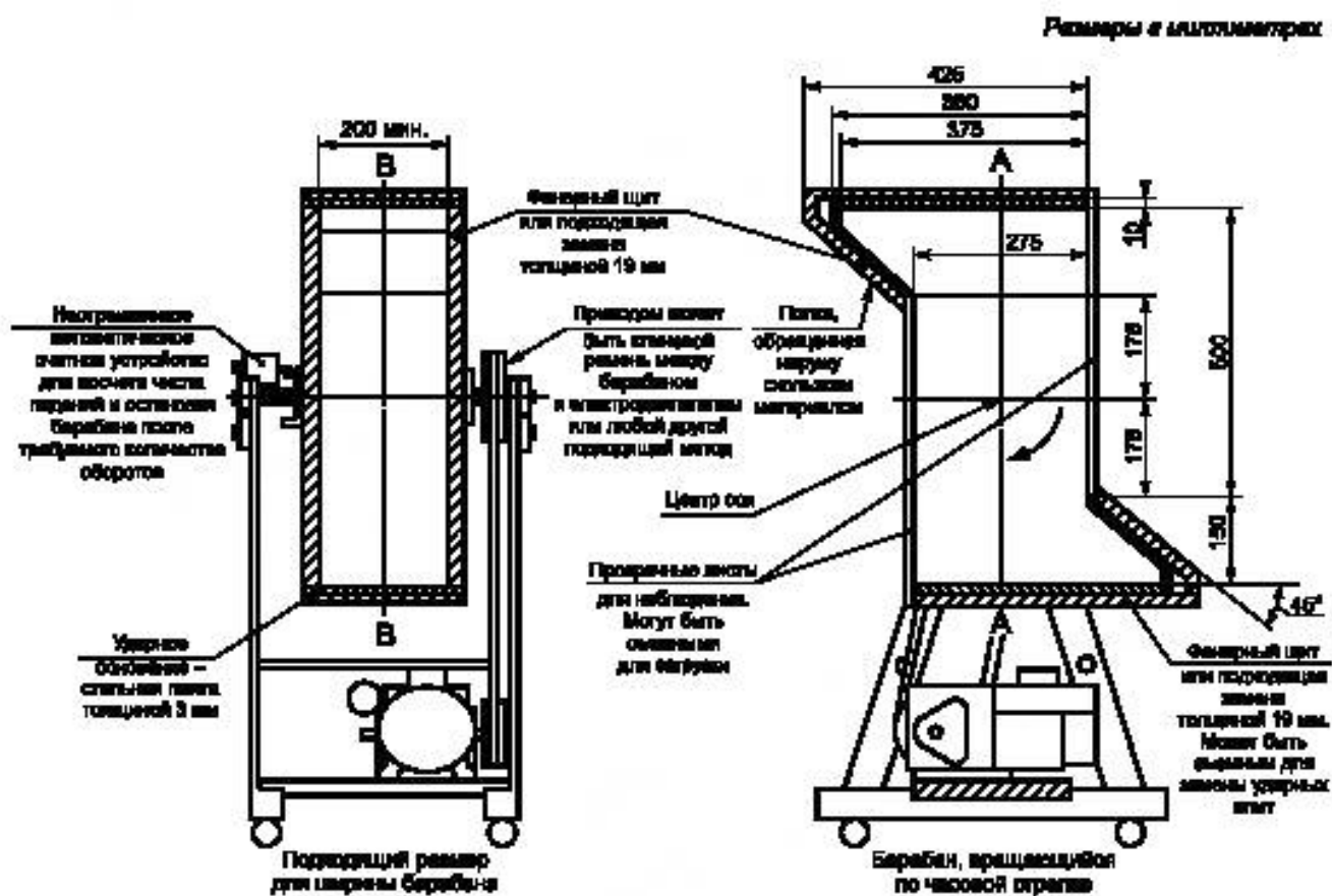
Рисунок 5 — Вращающийся барабан
