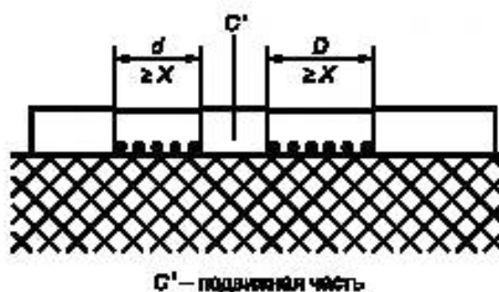
Рисунок В.9 — Узкое углубление
