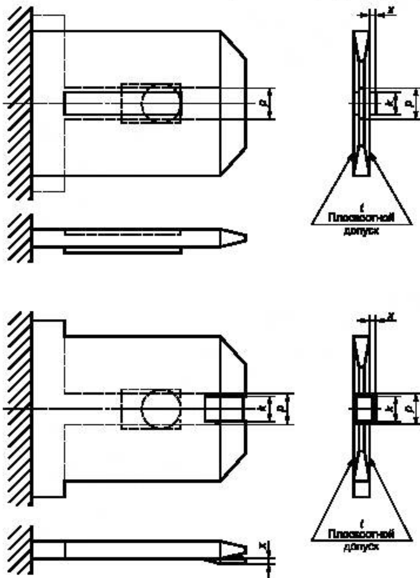
Рисунок 15 — Вставки для нереверсивных соединений
