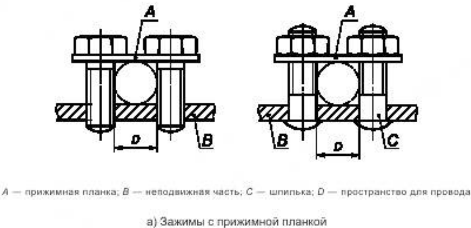
Рисунок 13 — Зажимы с прижимной планкой и под наконечник, лист 1
