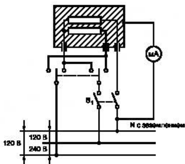
Рисунок 30 — Схема измерения тока утечки при рабочей температуре для двухфазного подключения управляющих устройств к трехпроводному питанию с заземленной нейтралью, за исключением управляющих устройств класса II
