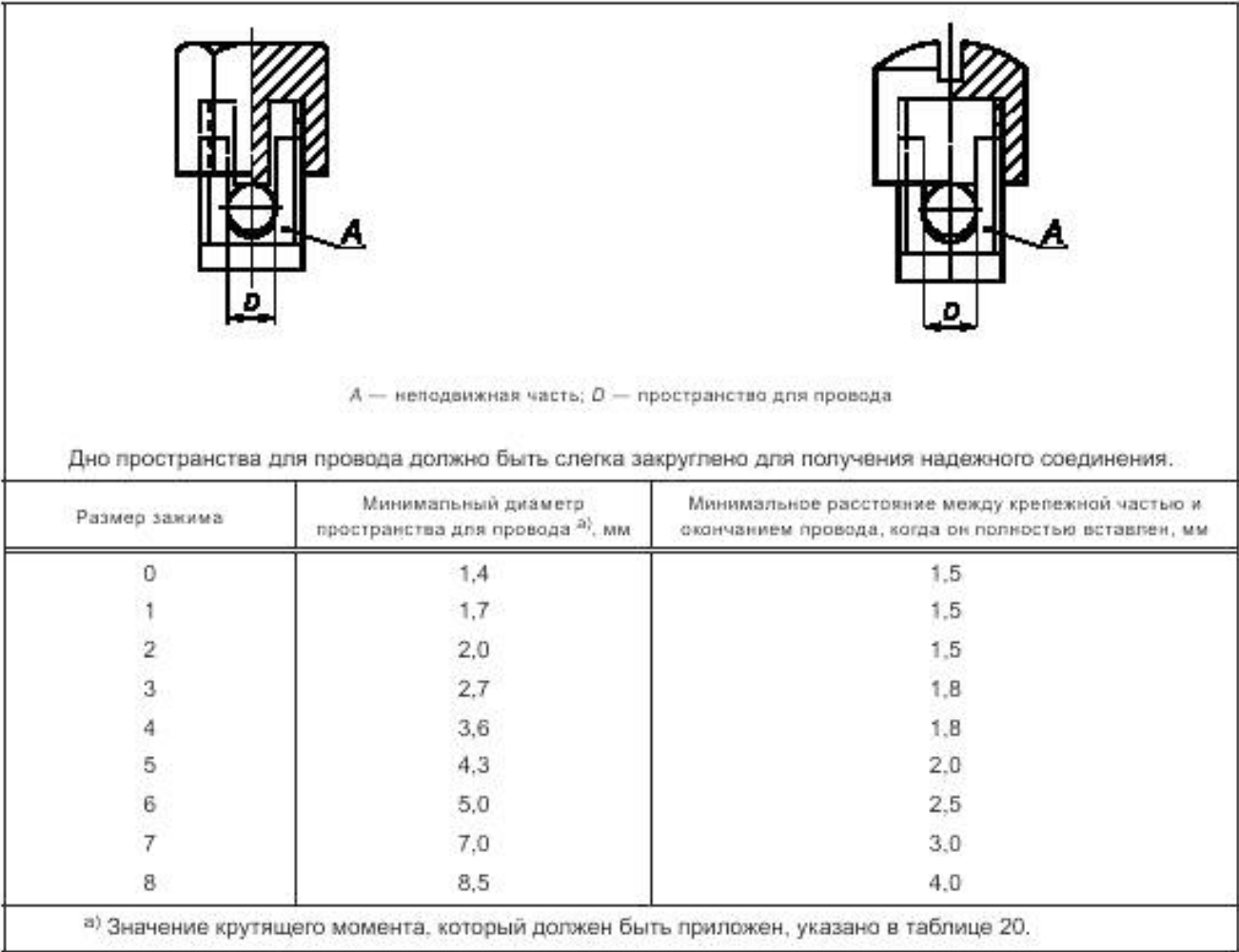
Рисунок 12 — Колпачковые зажимы
