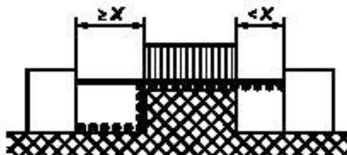
Рисунок В.6 — Несклеенное соединение с широкой прорезью
