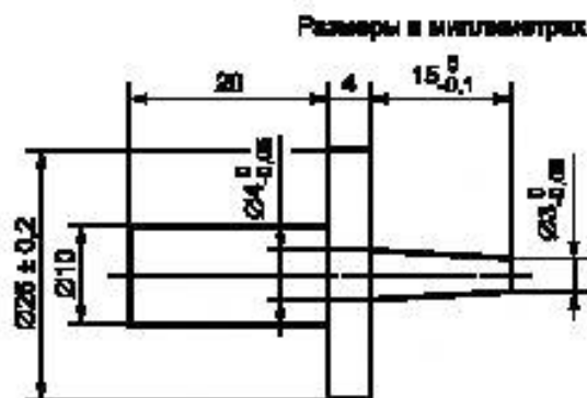
Рисунок 1 — Испытательный штырь
