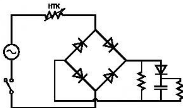
Рисунок J.1 — Испытательная цепь для испытания на износостойкость терморезистора, ограничивающего пусковой ток
