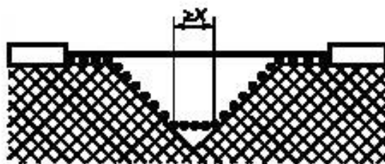
Рисунок В.2 — Широкая прорезь
