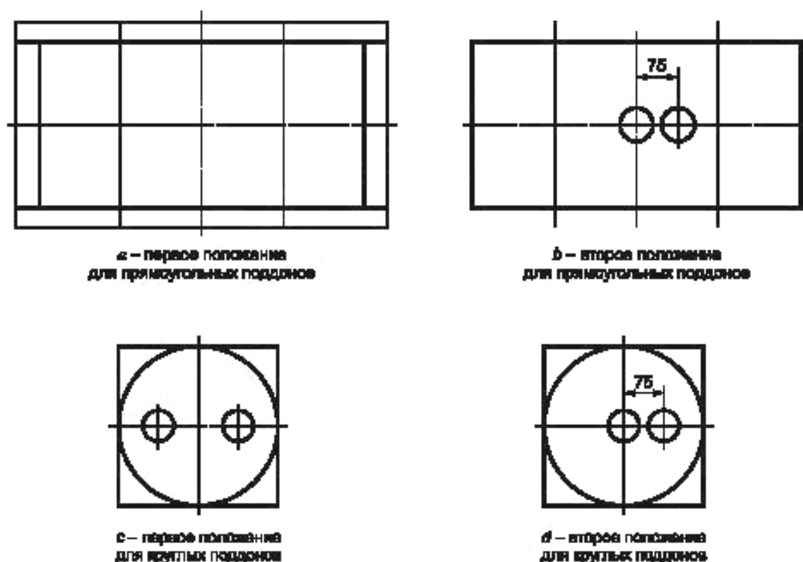
Рисунок 6 — Положение чаш для испытания по 11.1
