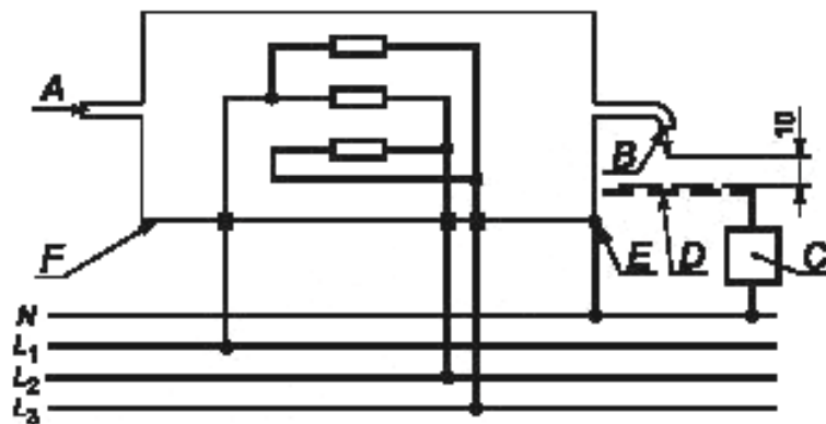
А — входное отверстие для воды; В — выходное отверстие для воды; С — схема на рисунке 4 IEC 60990; D — металлическая сетка; E — зажим заземления; F — корпус водонагревателя
