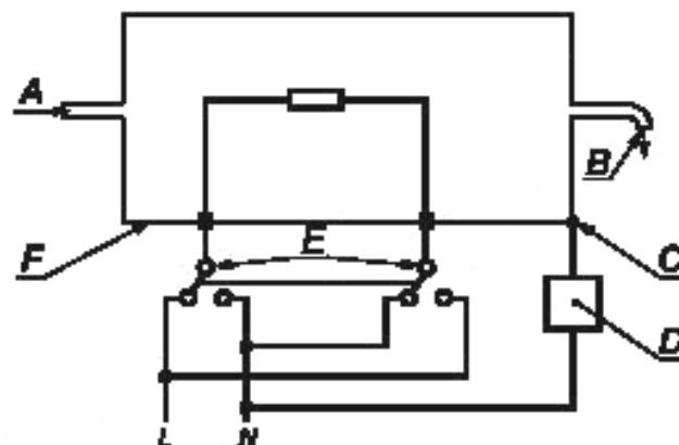
А — входное отверстие для воды; В — выходное отверстие для воды; С — зажим заземления; D — миллиамперметр; E — селективный переключатель; F — корпус водонагревателя
