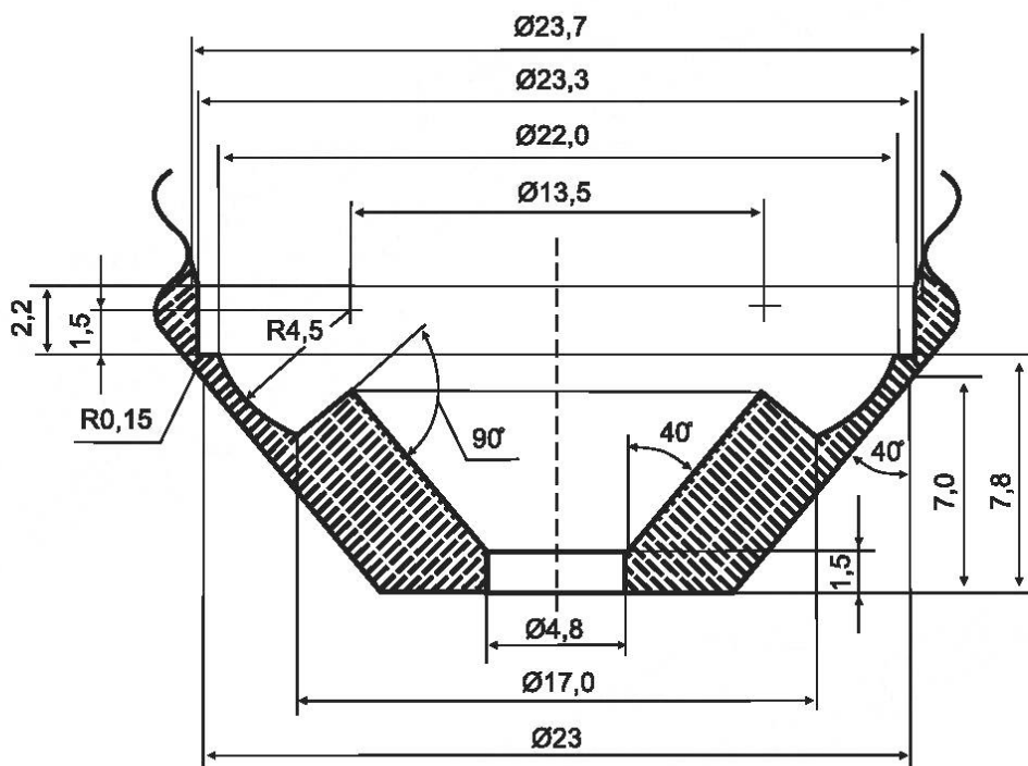
Предельные размеры цоколя E27
