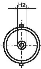
Остальные соответствуют размерам – как для BA15d
