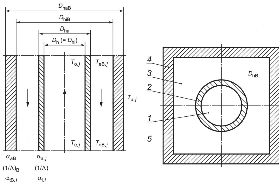
1 — дымоход (с дымовыми газами); 2 — шахта дымовых газов; 3 — воздушный тракт (с воздухом для горения); 4 — шахта воздуха; 5 — окружающий воздух
