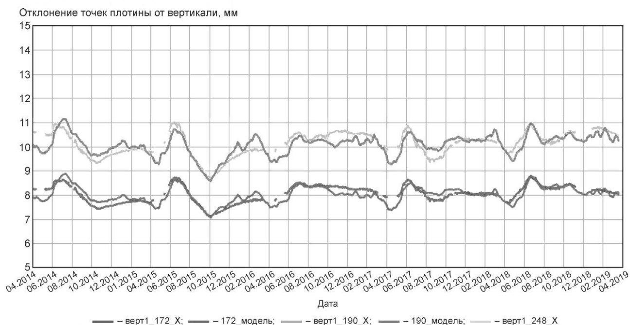
Рисунок Е.1 — Графики горизонтальных смещений станционной секции гравитационной бетонной плотины, построенные по данным натурных наблюдений по отвесам и полученные по прогнозным регрессионным моделям
