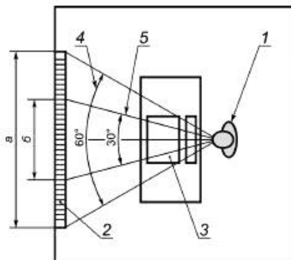
а — зона обзора; б — рабочая зона; 1 — оператор; 2 — внешний экран; 3 — экран дисплея АРМ; 4 — угол обзора экрана; 5 — угол обзора рабочей зоны экрана
