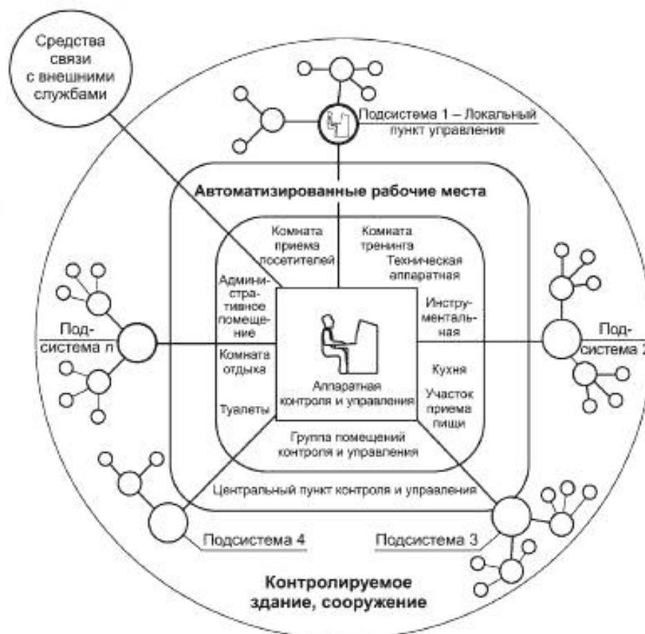
Рисунок А.1 — Обобщенная структурная схема ЦУКС
