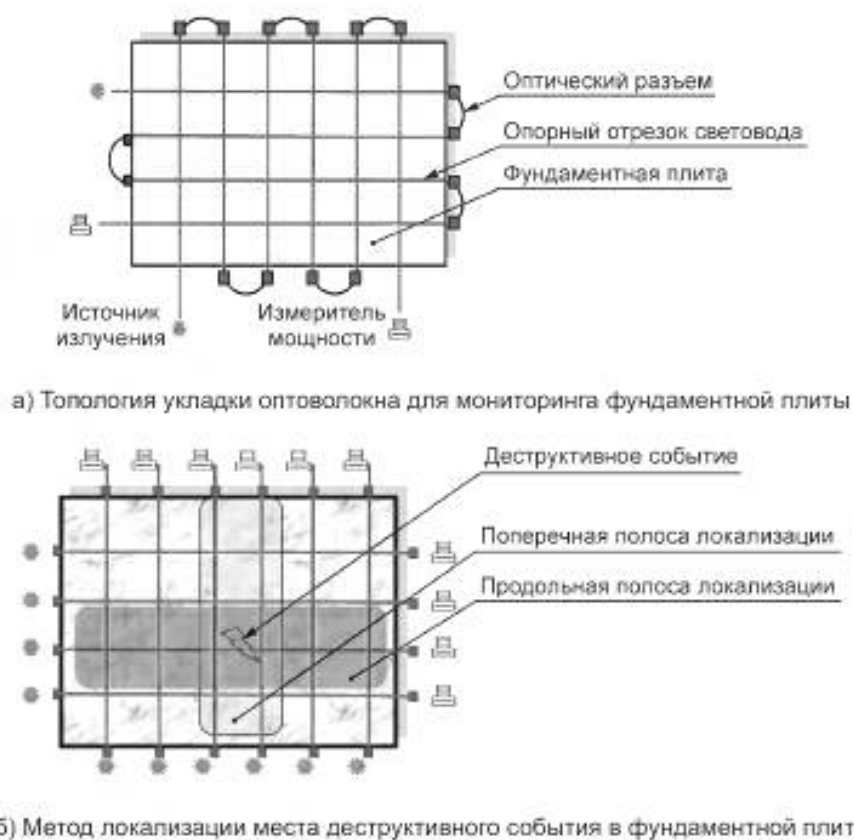
Рисунок 14 — Пример мониторинга деформаций в фундаментной плите с использованием оптоволокна
