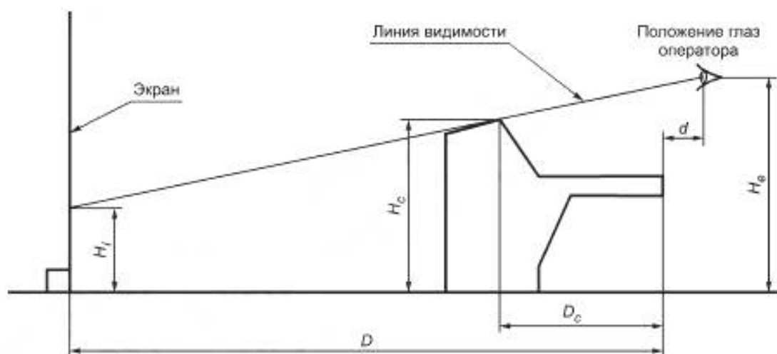
Рисунок А.4 — Элементы оборудования АРМ
