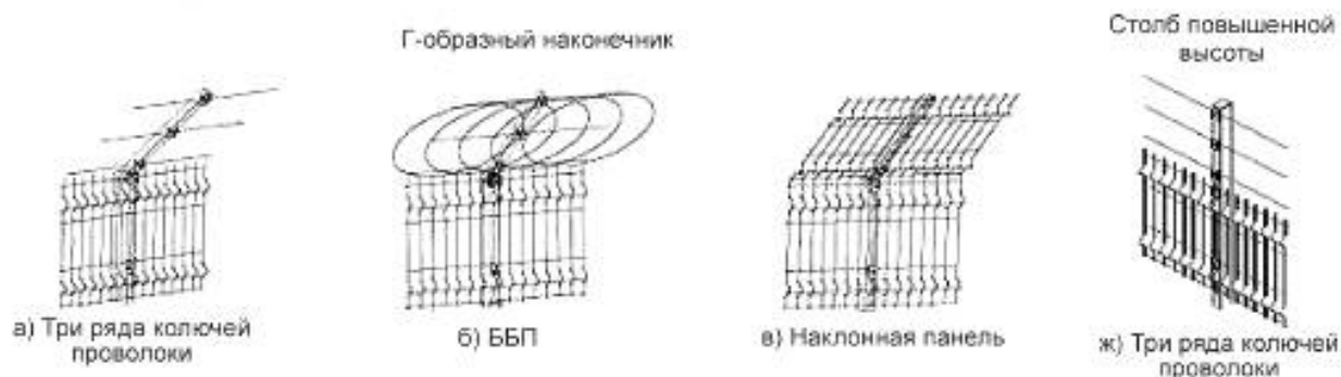
Рисунок 9, лист 1 — Варианты установки дополнительного верхнего ограждения
