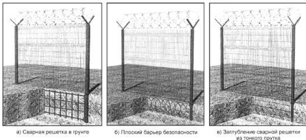
Рисунок 8 — Варианты выполнения нижнего дополнительного ограждения
