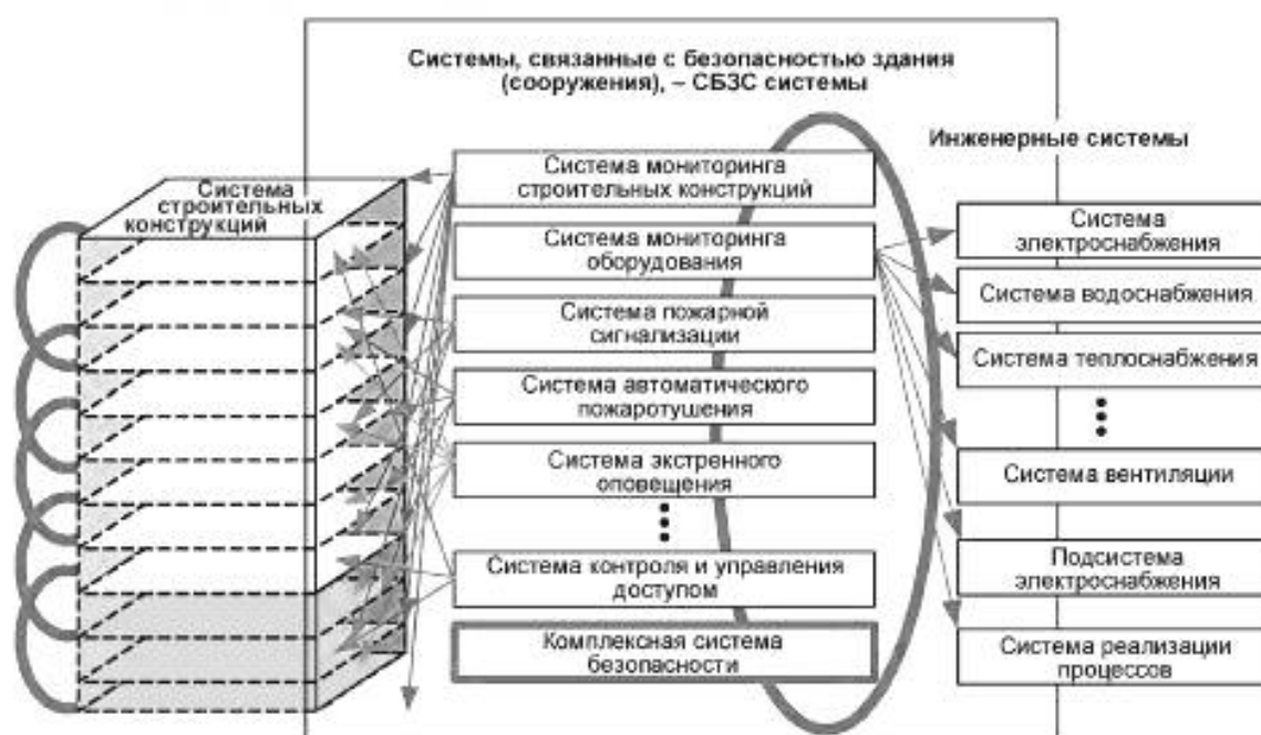
Рисунок 1 — Модель здания или сооружения как сложной системы
