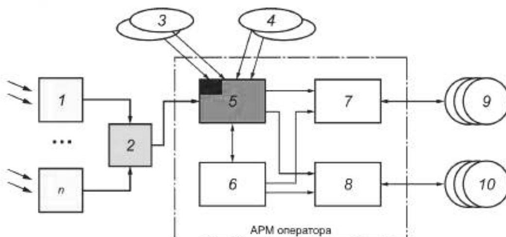
Рисунок 11, лист 1 — Обобщенная структурная схема системы мониторинга
