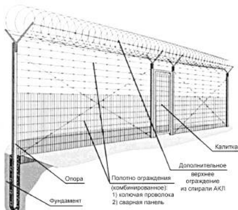
Рисунок 3 — Типовая конструкция и элементы защитного ограждения
