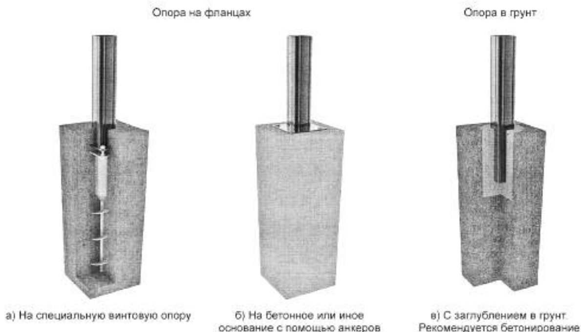
Рисунок 4 — Основные виды установки опор
