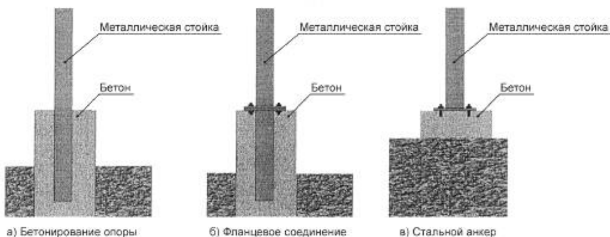
Рисунок 5 — Способы установки опор на железобетонный фундамент
