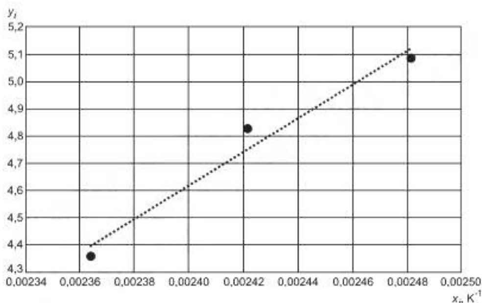
Рисунок 2 — Пример условного графика зависимости y_i от x_i
