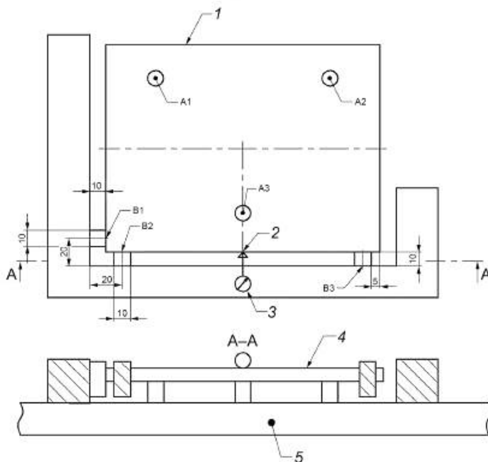
1 — панель; 2 — фронтальная крайка измерительного стержня индикатора диаметром 5 мм; 3 — индикатор часового типа; 4 — нижняя сторона панели; 5 — измерительный стол; A1...A3 — опоры, B1...B3 — поперечные упоры
