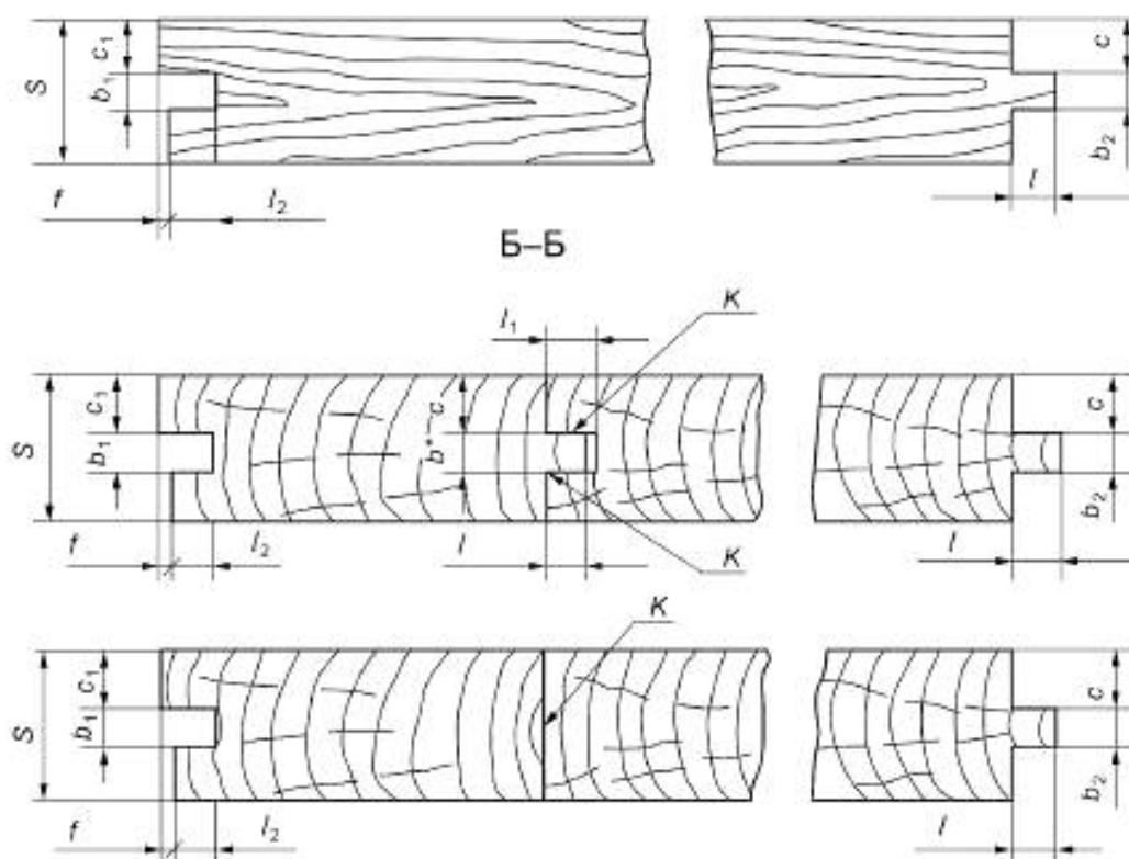
Рисунок 3 — Склейка кромок заготовок щита на гладкую фугу
