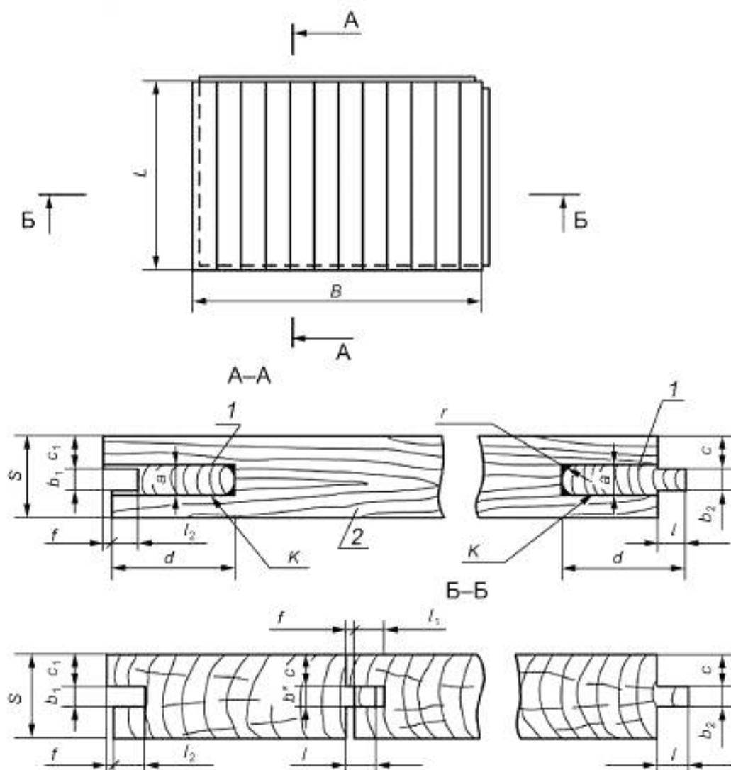
Рисунок 1 — Узел соединения щита с установленной шпонкой
