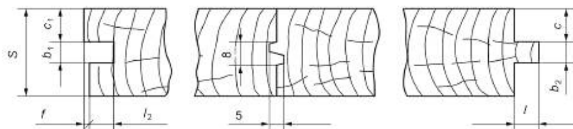
Рисунок 4 — Склейка кромок на продольный зубчатый шип
