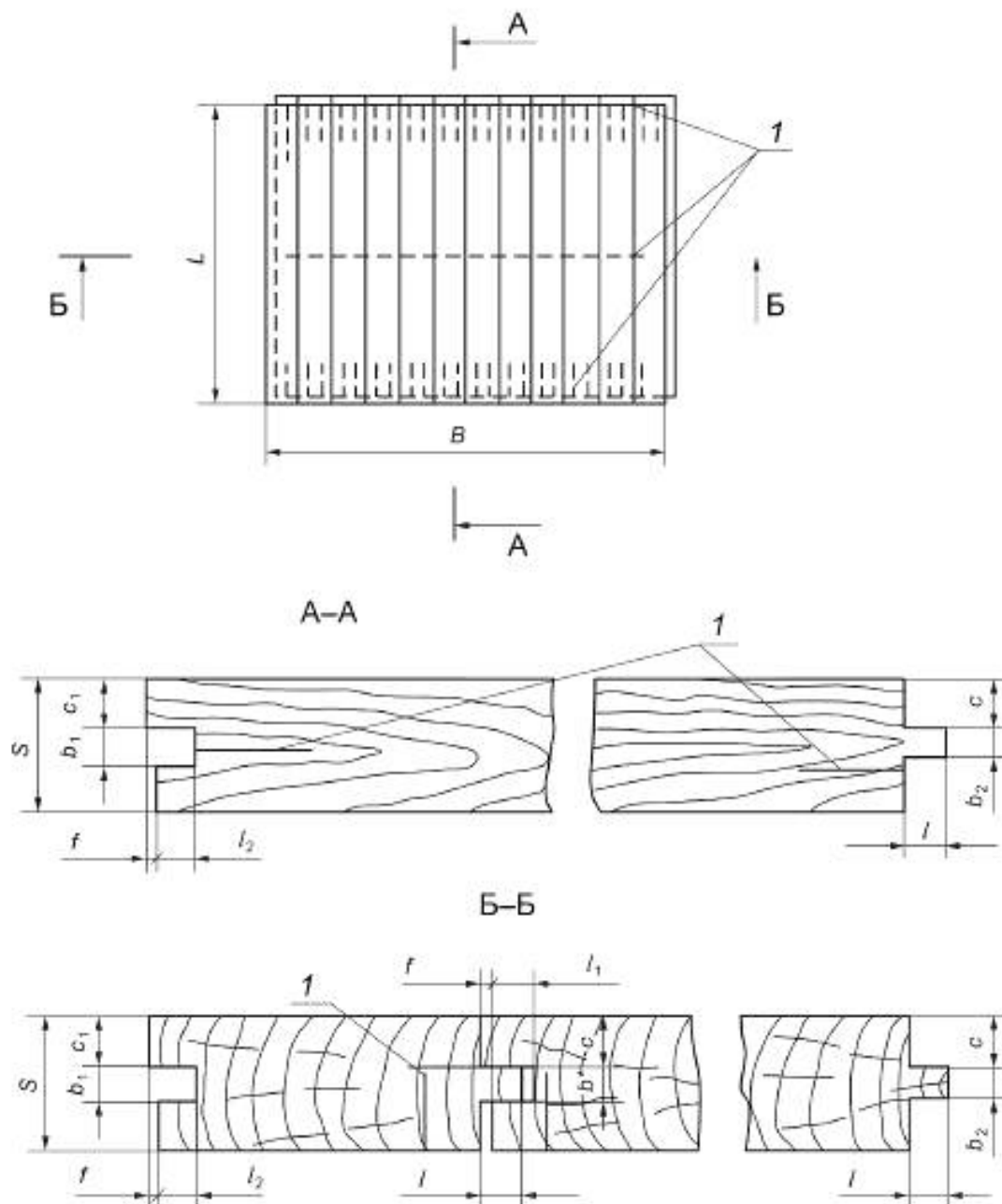
Рисунок 2 — Узел соединения щита, укрепленный П-образными скобами
