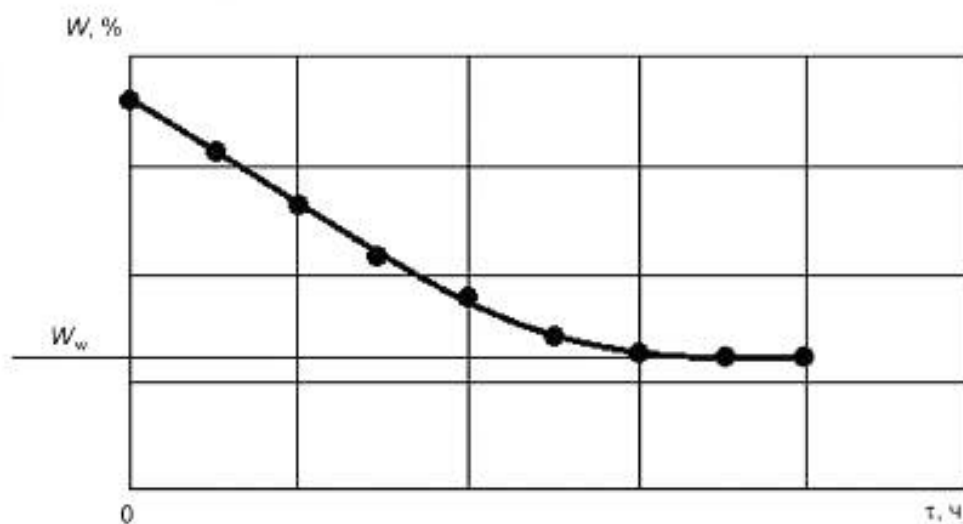
Рисунок А.2 — График изменения влажности грунта W над раствором электролита от времени экспозиции t
