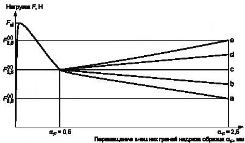
Рисунок В.4 — Характерный вид графика «нагрузка — перемещение внешних граней надреза образца» в зависимости от индекса подкласса сталефибробетона по остаточной прочности на осевое растяжение (а, b, c, d, e)
