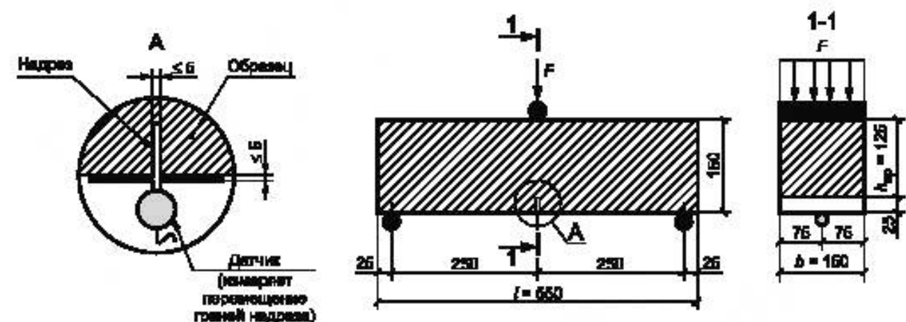
а — При измерении перемещения внешних граней надреза
