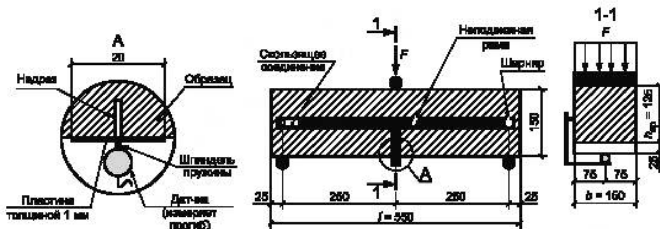
б — При измерении прогиба
