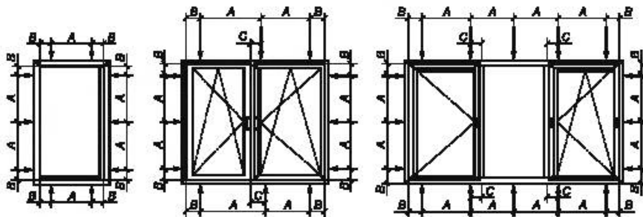
Рисунок В.10 — Схемы крепления оконных блоков
