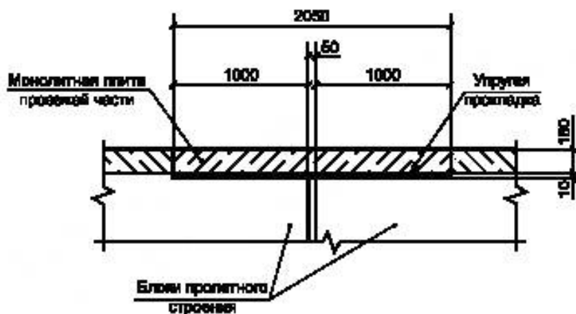
Рисунок В.2 — Схема отделенного участка соединительной плиты
