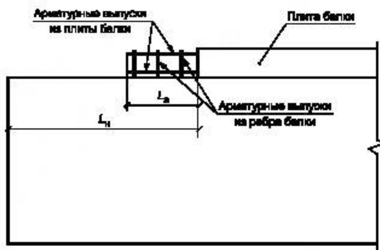
Рисунок А.1 — Балка с недобетонированной плитой
