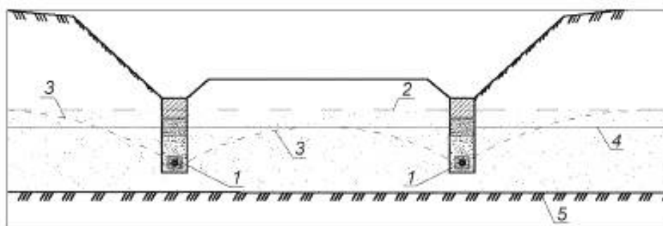
1 — дренажная труба с щебеночной засыпкой; 2 — уровень грунтовых вод до понижения; 3 — кривая депрессии после устройства дренажа; 4 — уровень грунтовых вод после понижения; 5 — водоупорный слой
