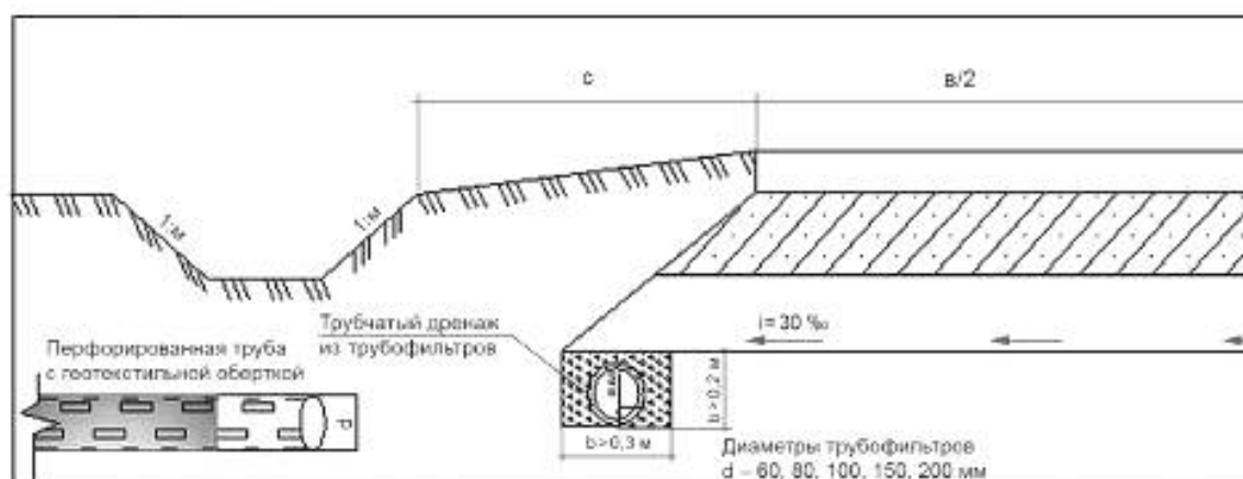
Рисунок 4 — Дренаж мелкого заложения из трубофильтров
