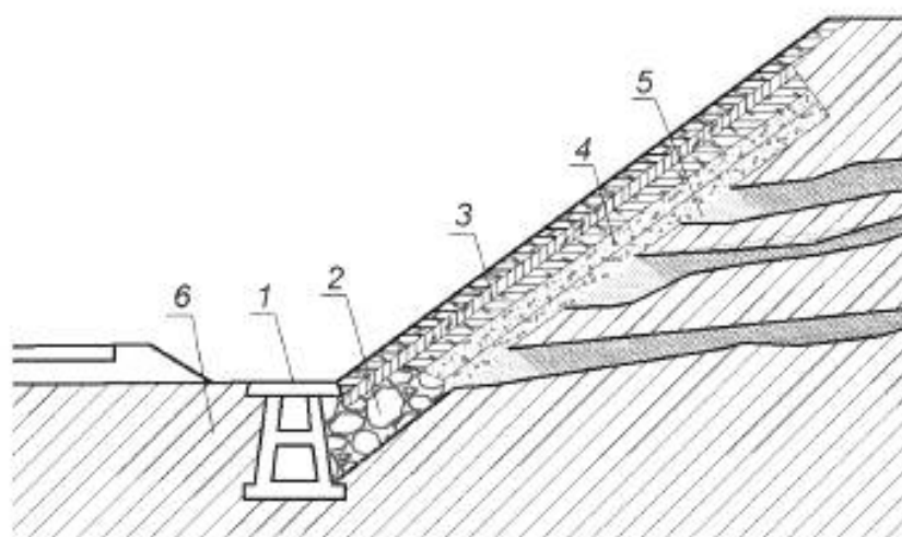
1 — железобетонный лоток; 2 — фильтр из крупнообломочного материала; 3 — одерновка; 4 — средний или крупный песок; 5 — водоносный песчаный слой; 6 — суглинок
