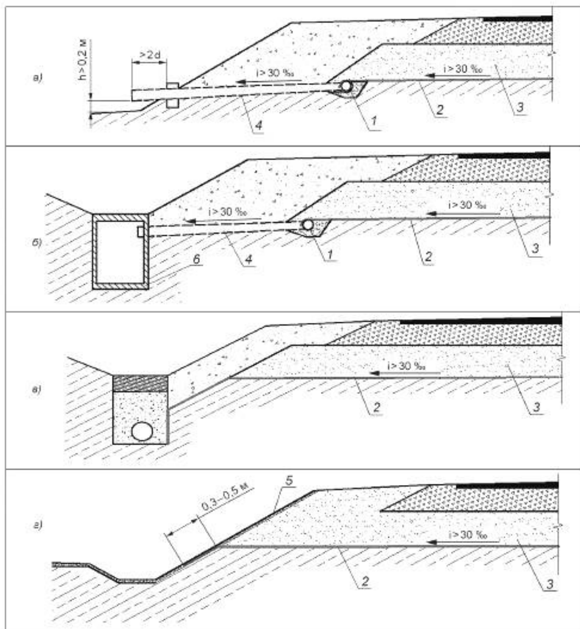
Дренажи с выпуском воды: а) — на рельеф; б) — в закрытый продольный лоток; в) — в трубчатый дренаж; г) — на откос насыпи 1 — продольная дренажная труба; 2 — геокomпозитный дренаж; 3 — песчаный дренирующий и технологический защитный слой с K_{\text{ф}} \geq 0,5 м/сут; 4 — дренажные трубы поперечных выпусков; 5 — растительный слой на откосе насыпи; 6 — закрытый продольный лоток
