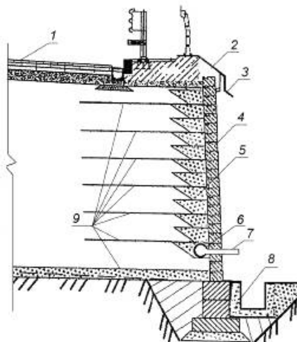
1 — автомобильная дорога; 2 — шалочный брус из бетона; 3 — козырек из листовой стали; 4 — стена из блоков; 5 — застенный дренаж из щебня в геотекстильной обертке; 6 — перфорированная труба продольного дренажа; 7 — водоотводная трубка; 8 — железобетонный полнок; 9 — слой геосетки
