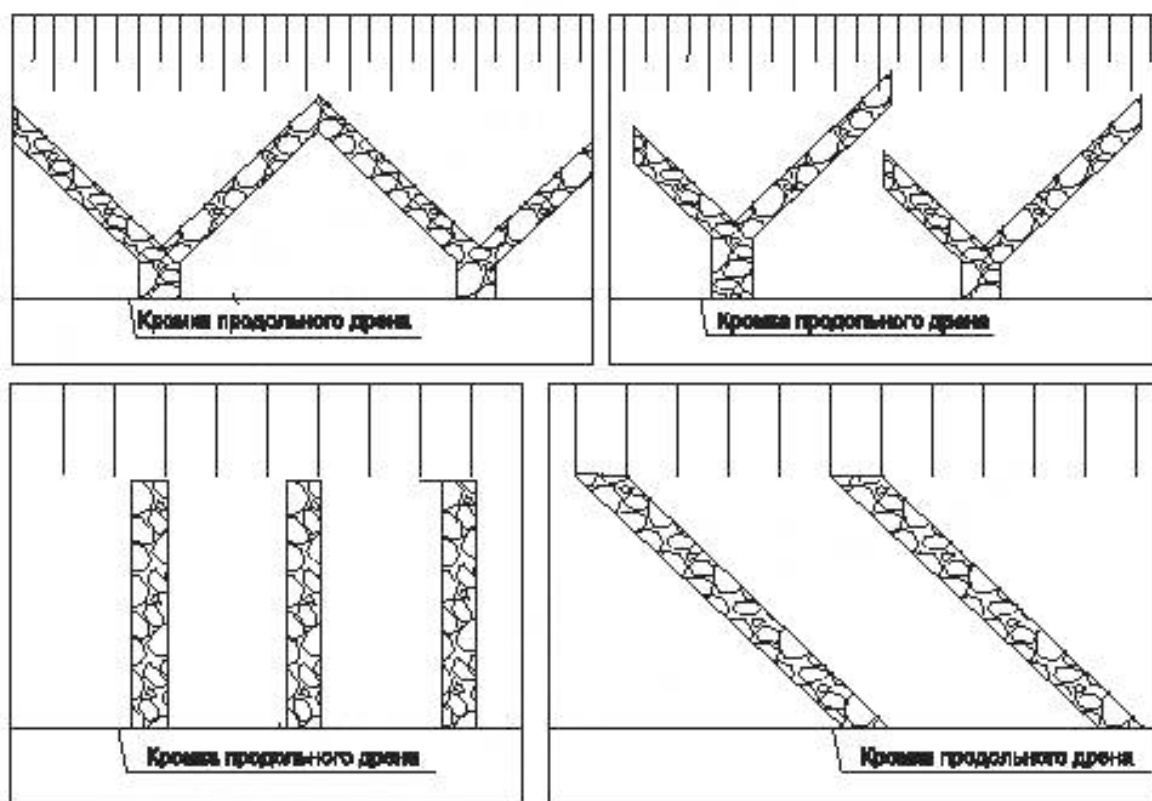
Рисунок 7 — Схемы размещения откосных дренажей в плане
