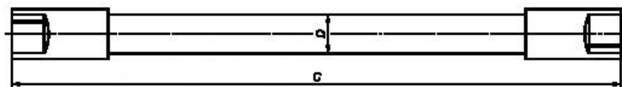
Цоколь W4.3x8.5d (см. лист 7004-115 ГОСТ IEC 60061-1)
