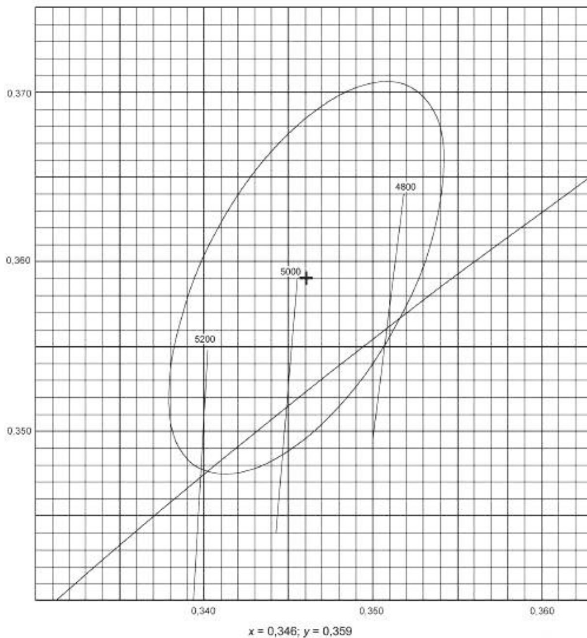
Рисунок D.2 — Площадь допусков для стандартной цветности F 5000
