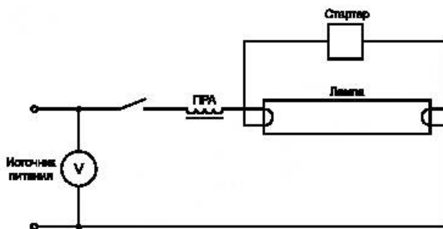
Рисунок А.1 — Схема испытания на зажигание ламп для работы со starterом
