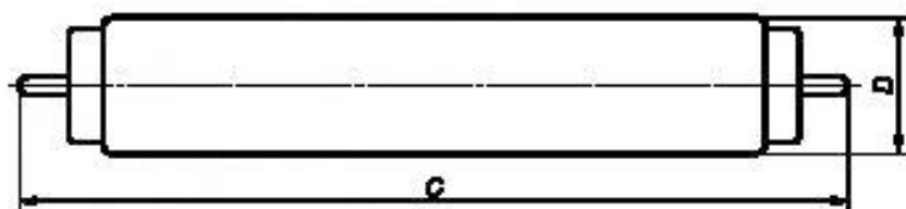
Цоколь Fa6 (см. лист 7004-55 ГОСТ IEC 60061-1)
