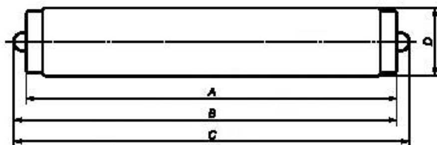
Цоколь Fa8 (см. лист 7004-57 ГОСТ IEC 60061-1)
