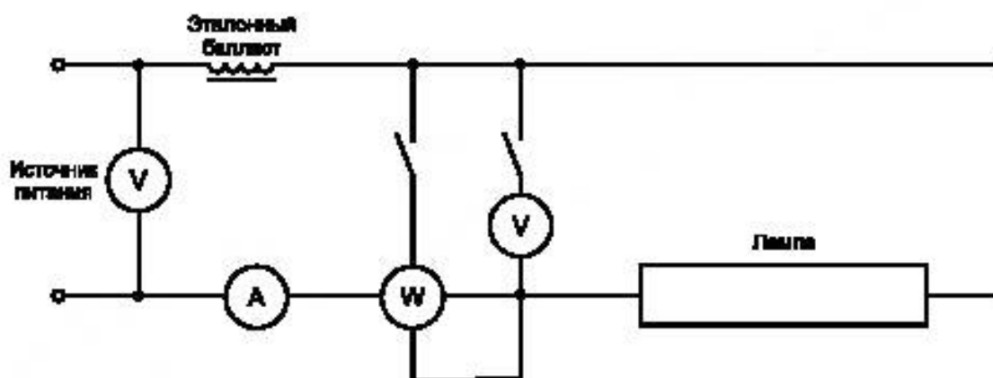
Рисунок В.3 — Схема измерения электрических и световых параметров ламп без предварительного подогрева катодов
