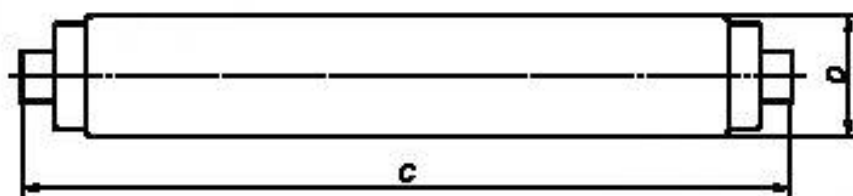
Цоколь R17d (см. лист 7004-56 ГОСТ IEC 60061-1)
