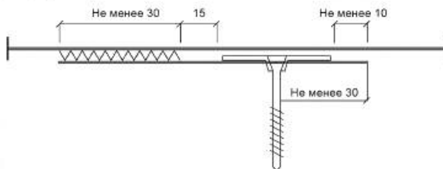
Рисунок 9 — Установка телескопического крепежа по краю рулона
