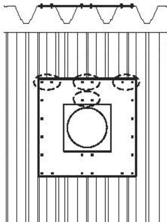
Рисунок 1 — Усиление сквозных проходов коммуникаций листом оцинкованной стали
