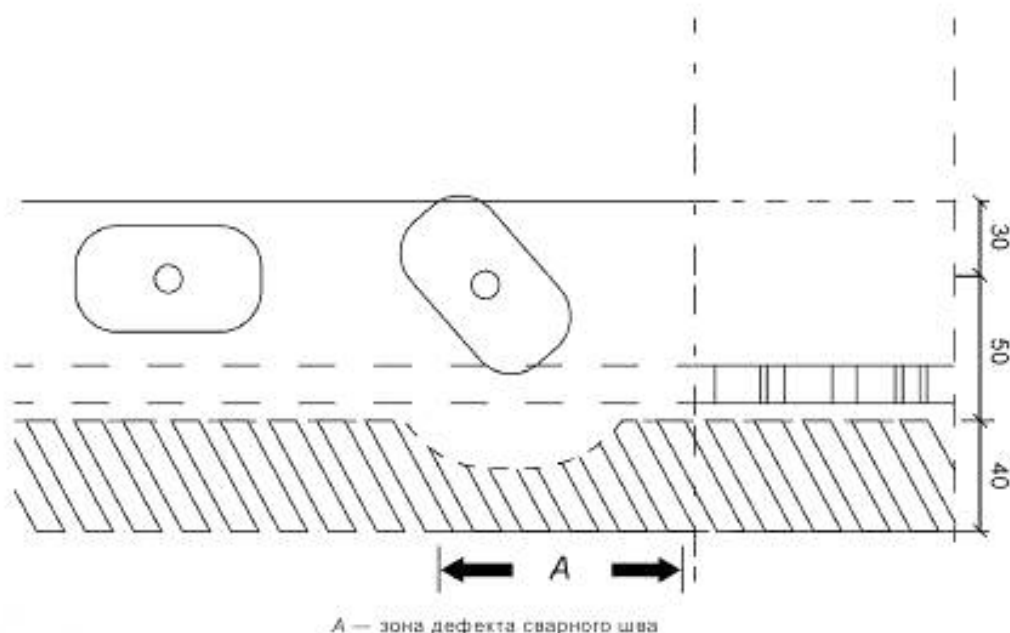
Рисунок 10 — Установка тарельчатого крепежа с овальной шайбой по краю полотна
