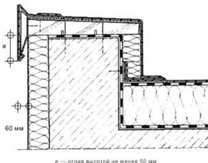
Рисунок 13 — Установка отлива по внешнему краю парапета
