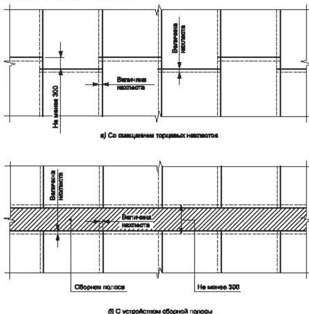
Рисунок 8 — Варианты раскладки кровельных рулонных полимерных материалов
