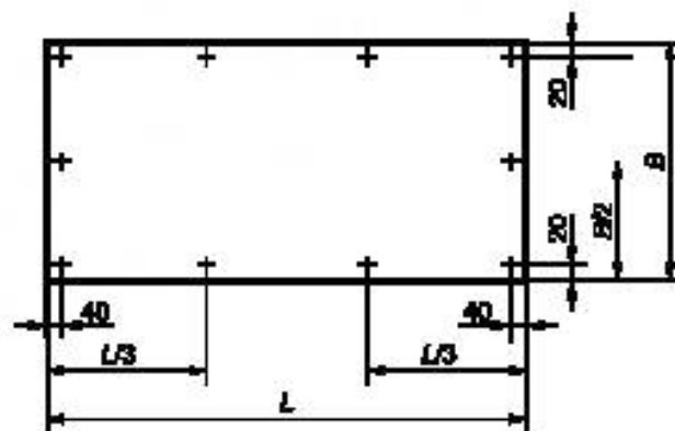
Рисунок 2 — Схема расположения точек измерения толщины АКЛ
