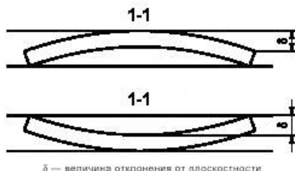
Рисунок 4 — Схема проверки АКЛ на отклонение от плоскостности
