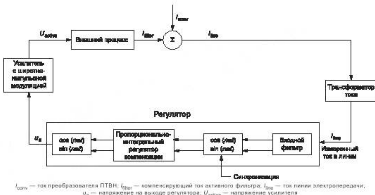
Рисунок 8 — Система управления активным фильтром с обратной связью
