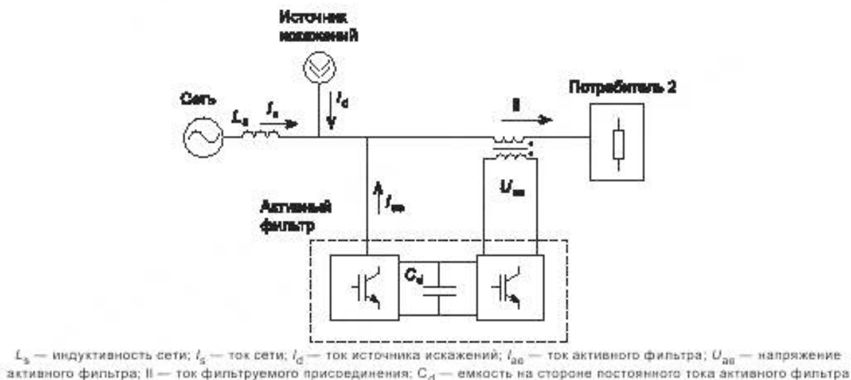
Рисунок 4 — Подключение параллельно-последовательного активного фильтра
