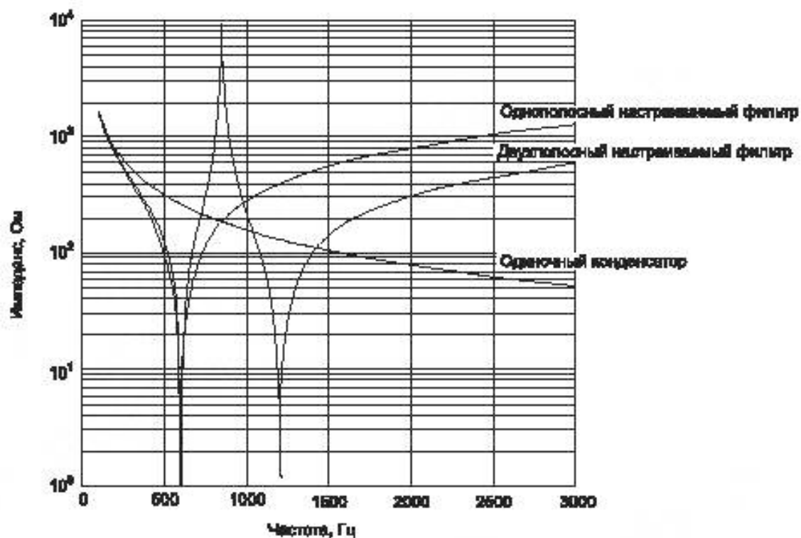
Рисунок А.1 — Характеристики импеданса различных пассивных фильтров
