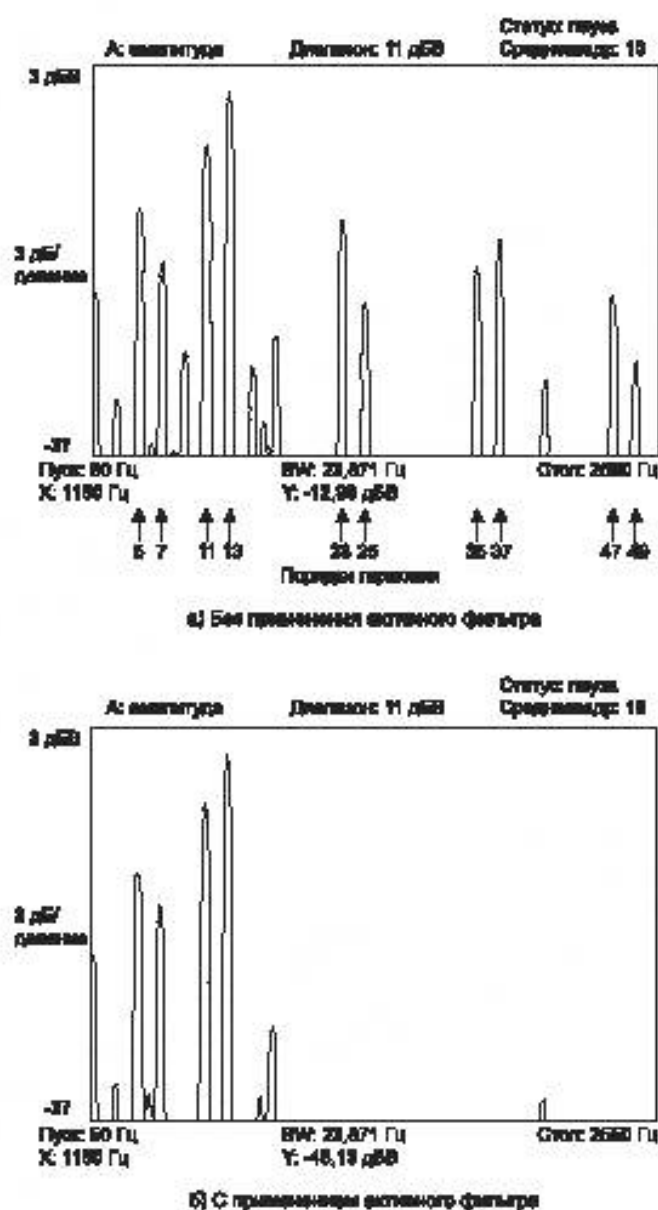
Рисунок В.1 — Графики по результатам полевых измерений
