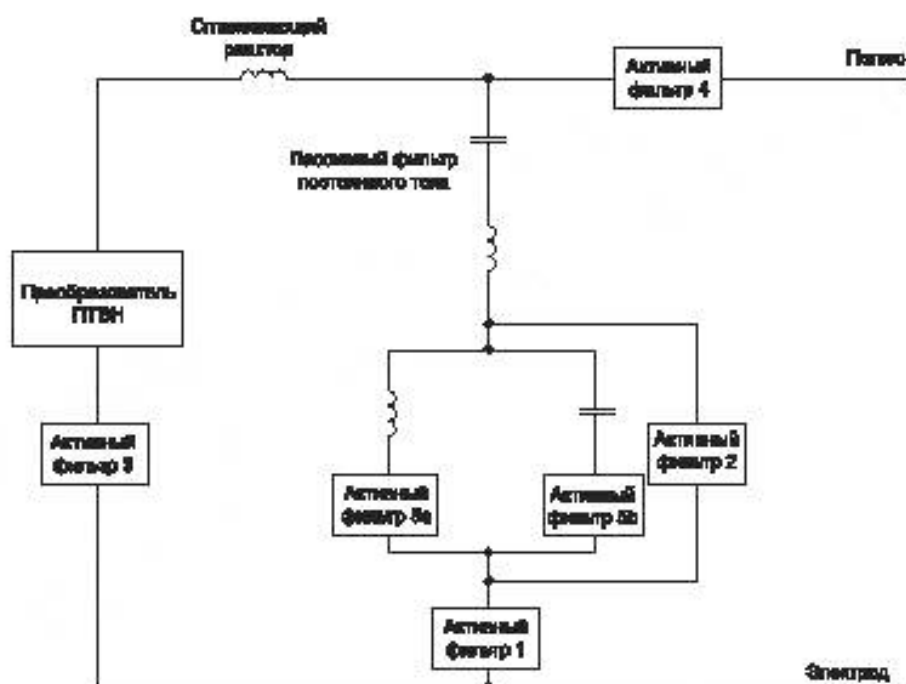
Рисунок 5 — Варианты подключения активных фильтров постоянного тока
