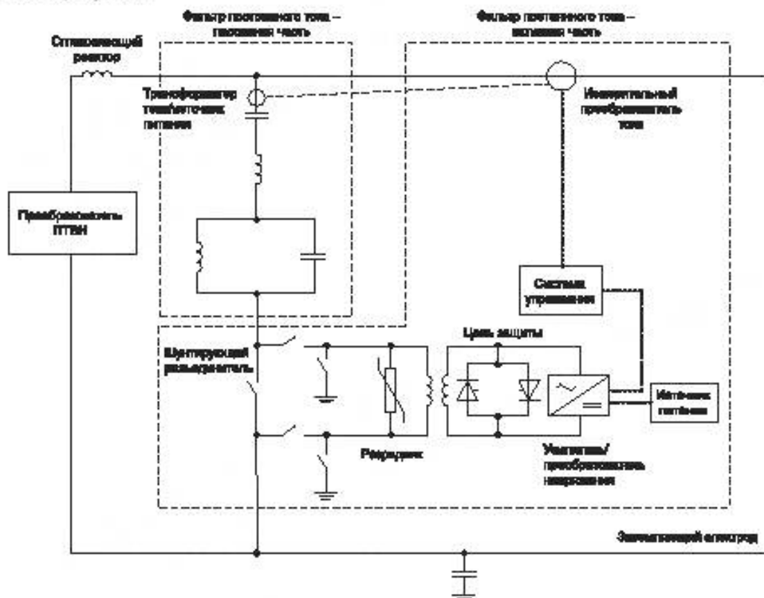
Рисунок 6 — Компоненты активного фильтра постоянного тока
