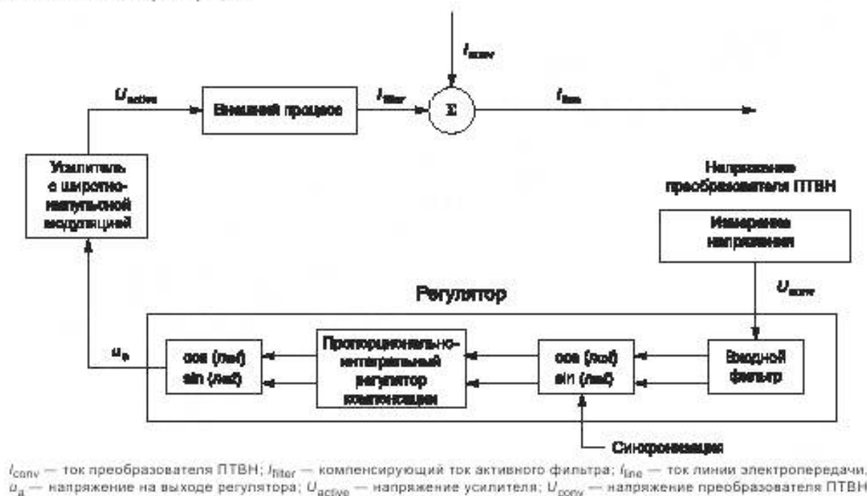
Рисунок 7 — Структурная схема системы управления активным фильтром с прямой связью
